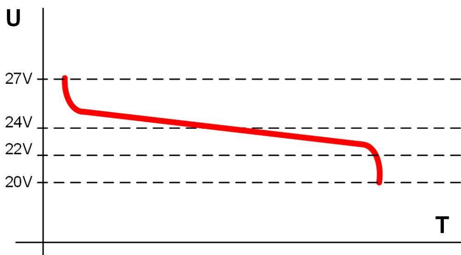
Рисунок 3.11.3 – Снижение напряжения при разрядке АКБ.
