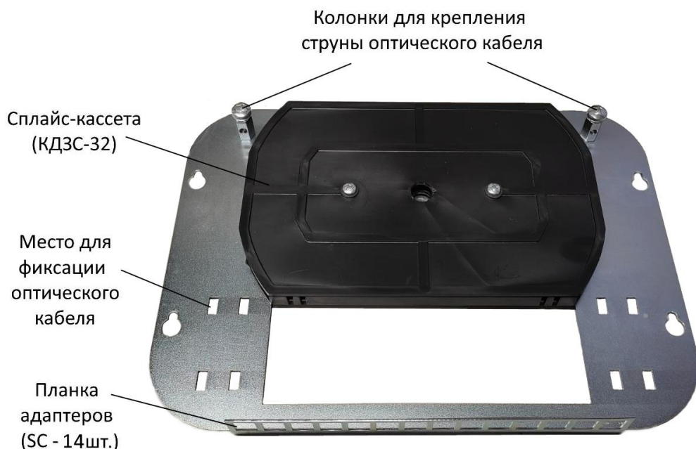
Рисунок 3.3.1 - Оптический кросс.
