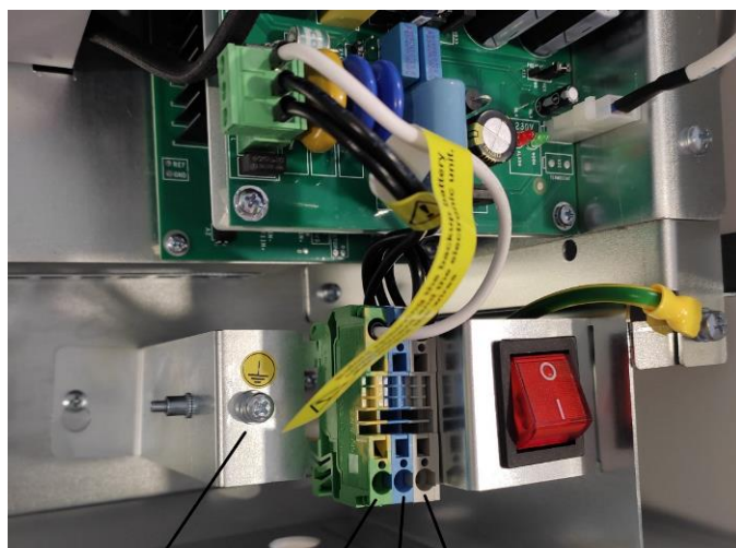
Рисунок 3.5.1 – Узел подключения питания.
