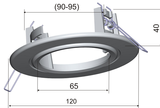
Рис.1. Габаритные и установочные размеры
