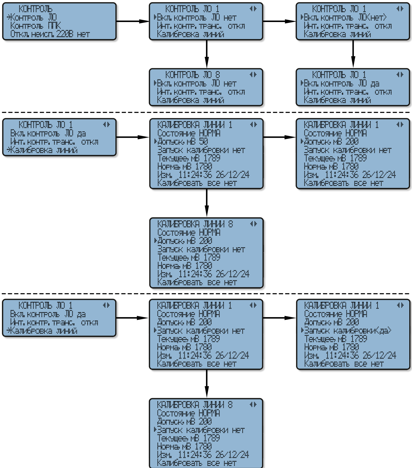
Рисунок 34. Калибровка, включение / отключение контроля ЛО.
