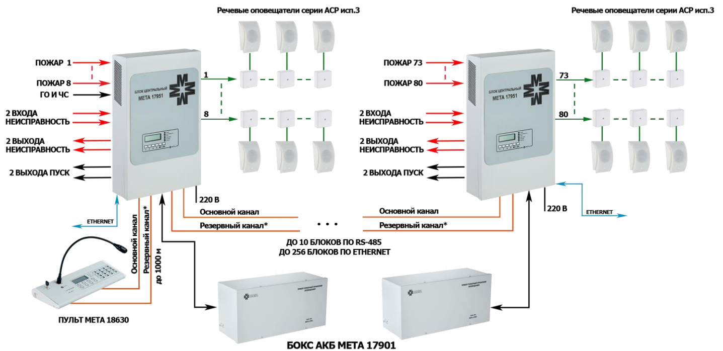
Рисунок 11. Структурная схема СОУЭ на 80 зон, построенная на базе ЦБ МЕТА 17950/17951.
