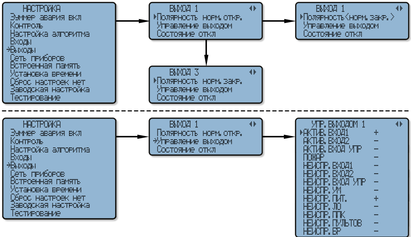
Рисунок 37. Настройка клемм Выход 1, Выход 2, Выход 3.
