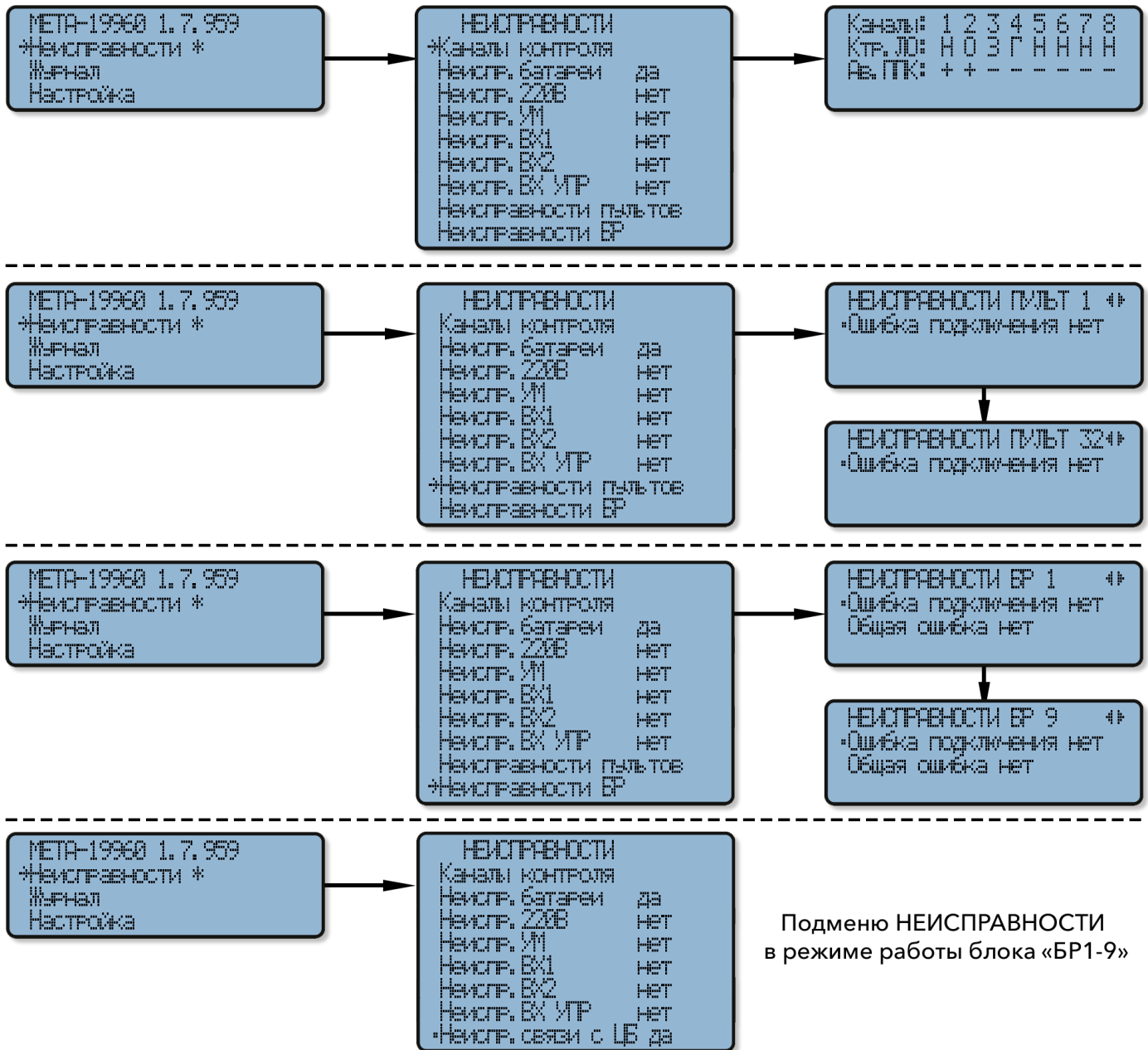
Рисунок 40. Окно НЕИСПРАВНОСТИ.
