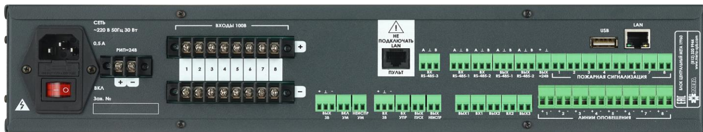
Рисунок 4. Расположение элементов коммутации (клемм и разъемов) на задней панели ЦБ МЕТА 19960.
