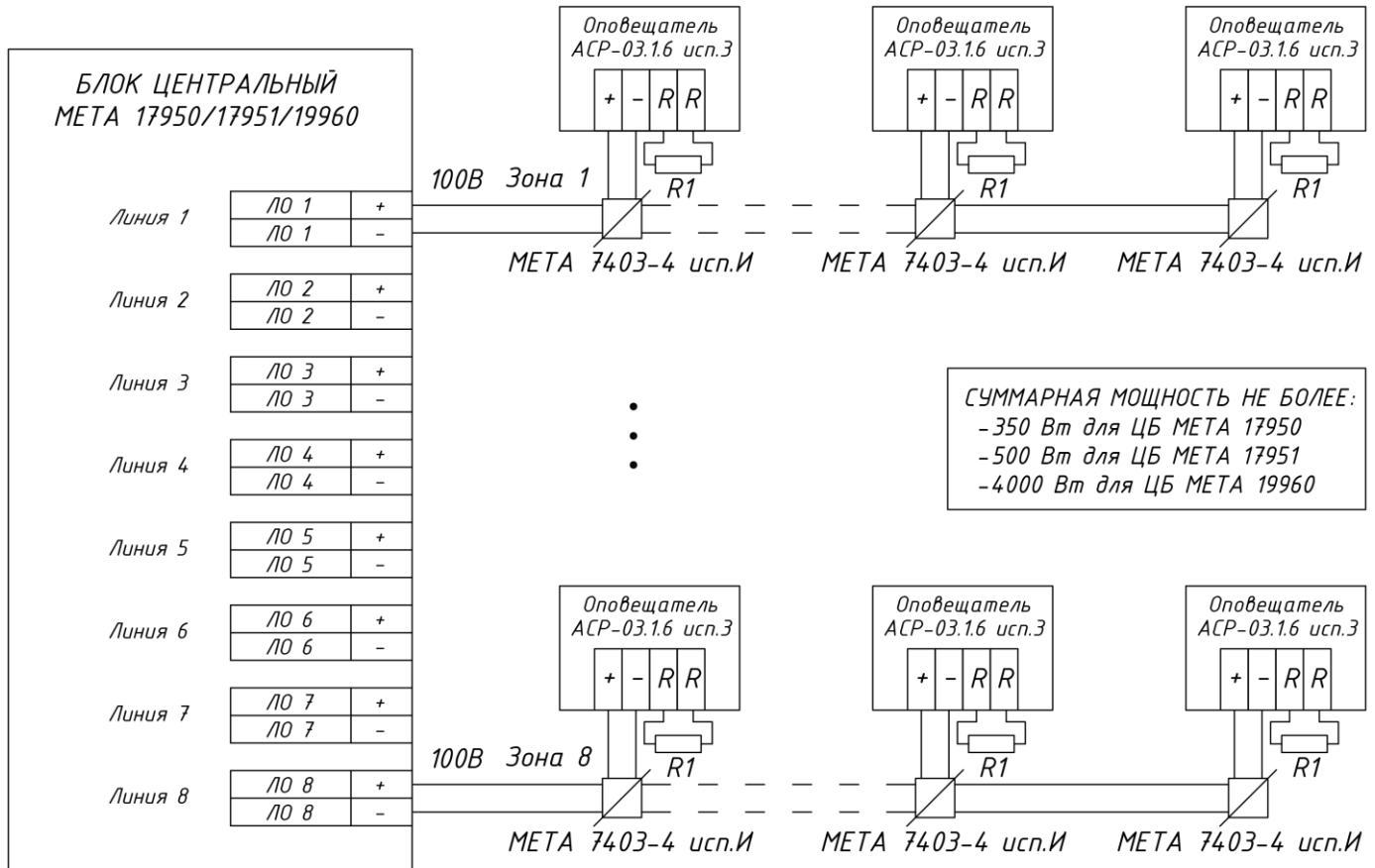
Рисунок 18. Схема подключения речевых оповещателей на ЛО.
