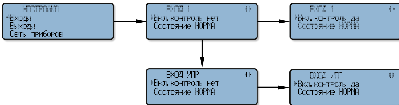
Рисунок 33. Включение / отключение контроля клемм «ВХ. УПР».
