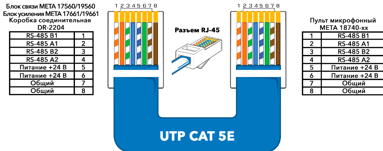
Рисунок 25. Схема подключения кабеля от БС МЕТА 17560/19560, БУ МЕТА 17661/19661 или соединительной коробки DR-2204 к МП МЕТА 18740-хх.
