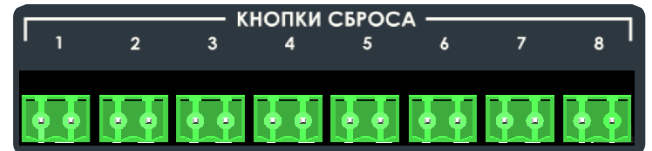
Рисунок 34. Клеммы «ВХОД КНОПКИ СБРОСА 1 – 8» для подключения УС МЕТА 7520 к БС МЕТА 19560.
