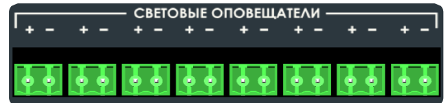
Рисунок 36. Клеммы «ВЫХОД СВЕТОВЫЕ ОПОВЕЩАТЕЛИ 1 – 8» для подключения табло МЕТА 7523 и МЕТА 7523 исп.1 к БС МЕТА 19560.
