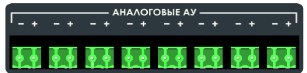
Рисунок 30. Клеммы «ВЫХОД АНАЛОГОВЫЕ АУ 1 – 8» для подключения АУ к БС МЕТА 19560.
