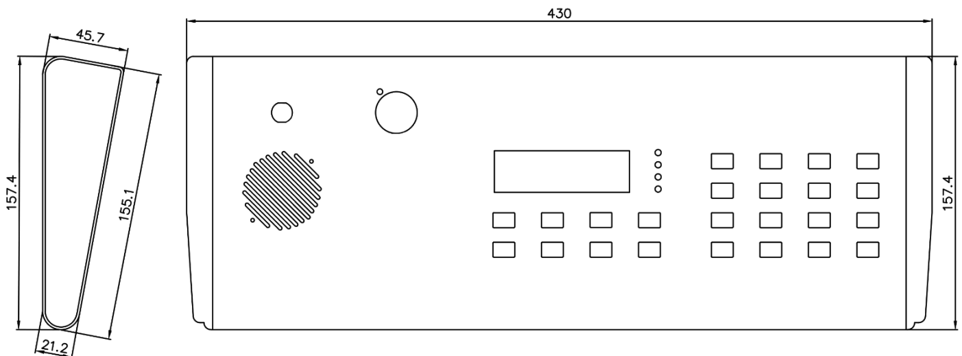
Рисунок 2. Габаритные размеры МП МЕТА 18740-16.
