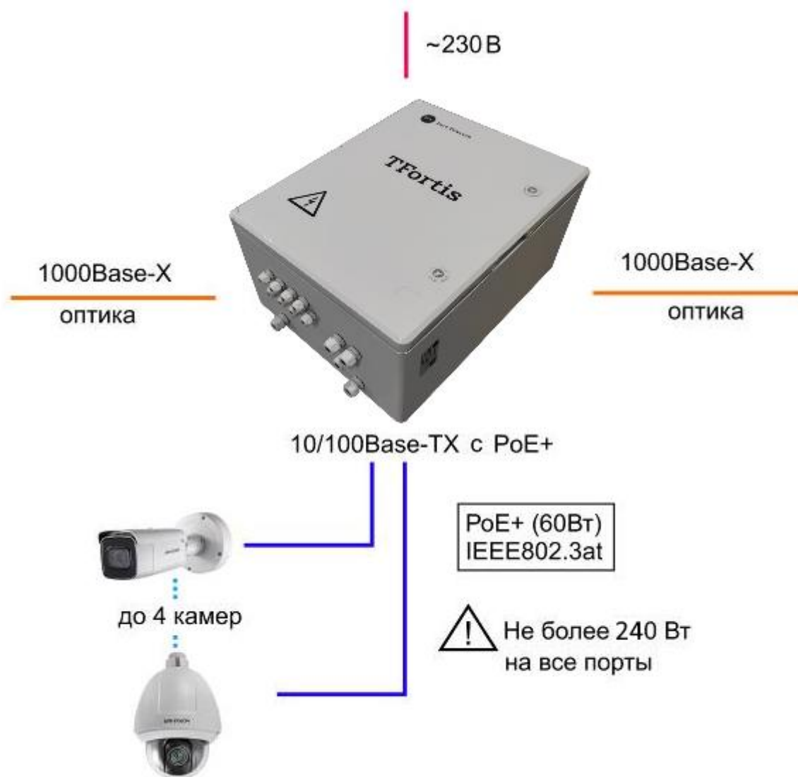
Рисунок 1 - Схема подключения PSW-2G+UPS-Box
