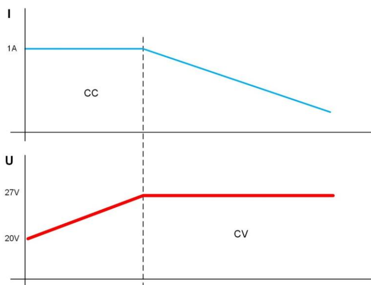
Рисунок 3.11.2 – Зависимость постоянного тока и напряжения заряда АКБ.
