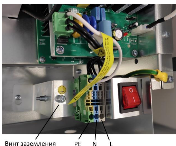
Рисунок 3.5.1 – Узел подключения питания.
