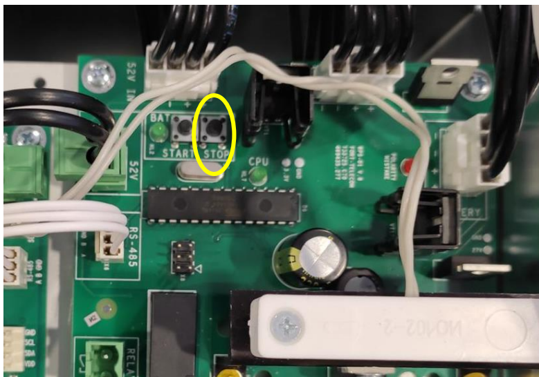
Рисунок 3.5.3 – Нажмите и удерживайте кнопку STOP в течение 5 сек. для отключения питания от АКБ.
