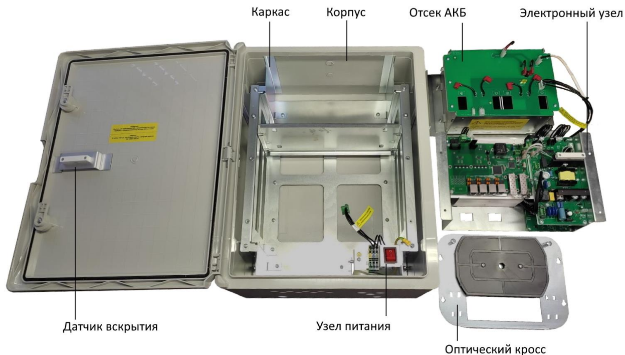
Рисунок 3.1.3 – Основные элементы коммутатора
