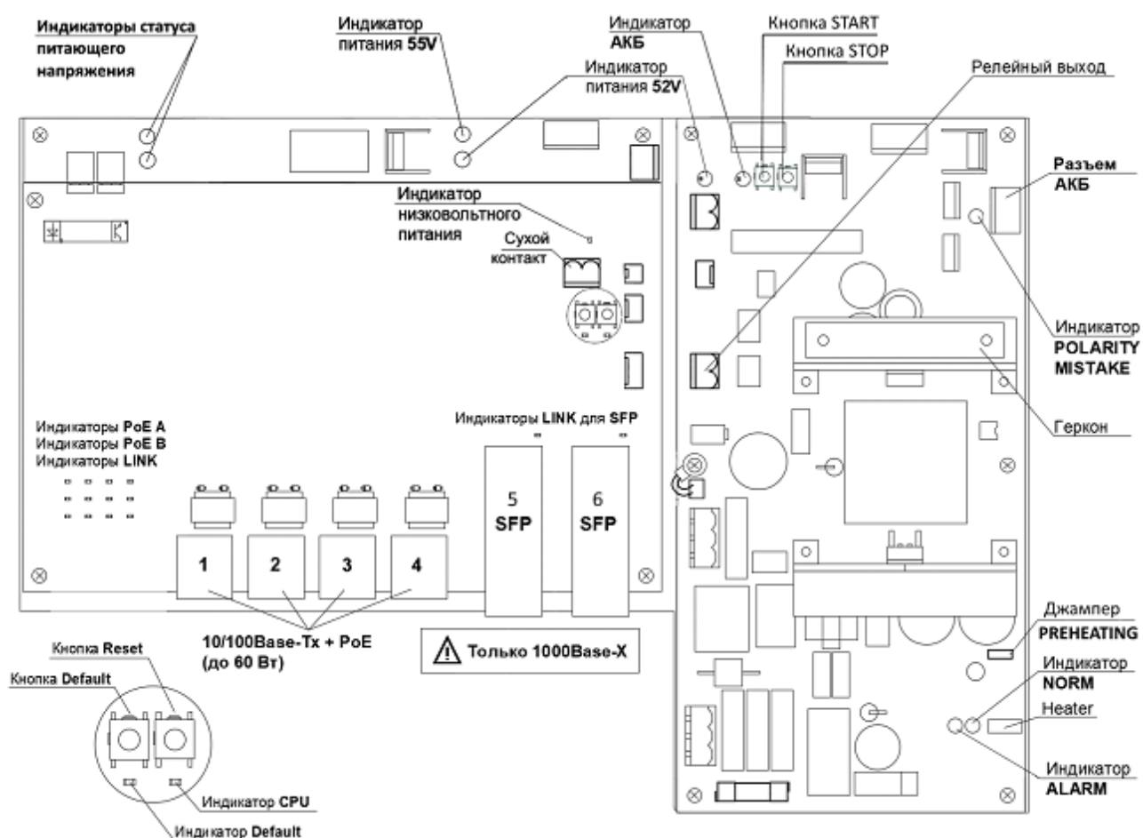
Рисунок 3.4.1 – Расположение элементов PSW-2G+UPS-Box
