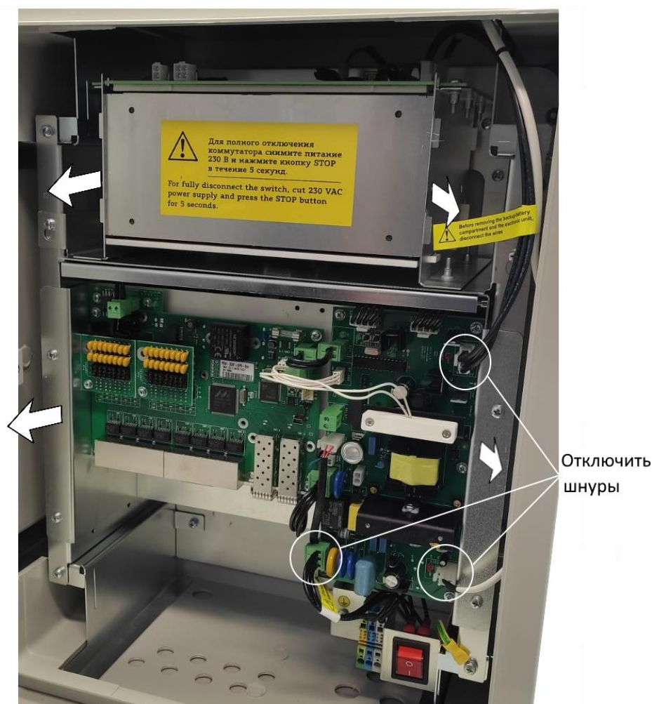
Рис. 7.1.1. Извлечение отсека АКБ и электронного узла
