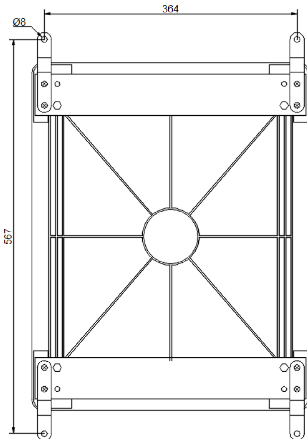
Рисунок 7.2 - Разметка крепления
