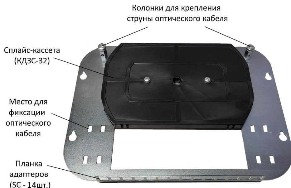
Рисунок 3.3 - Оптический кросс.
