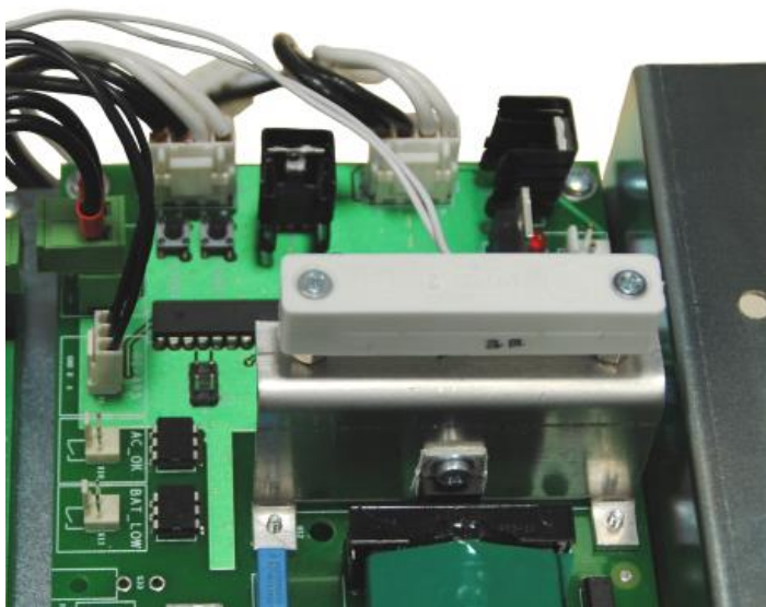
Рисунок 3.7.2 - Датчик вскрытия в корпусе коммутатора
