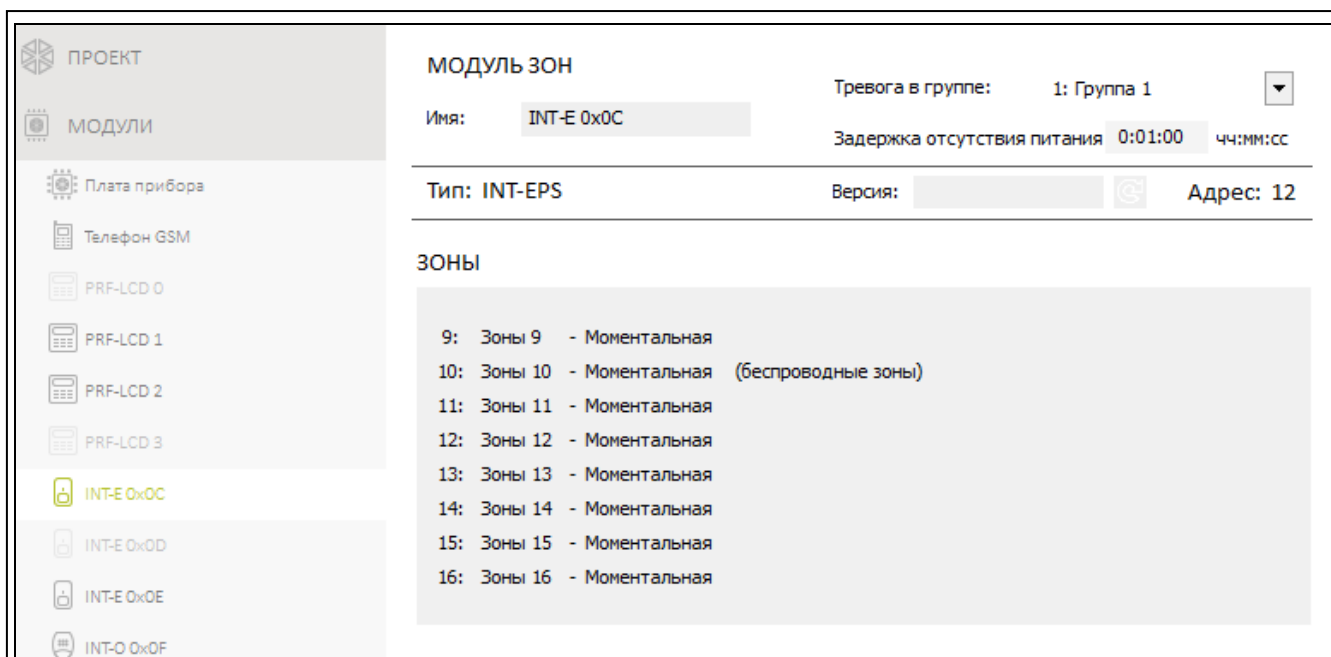
Рис. 11. Закладка с установками модуля расширения зон.
