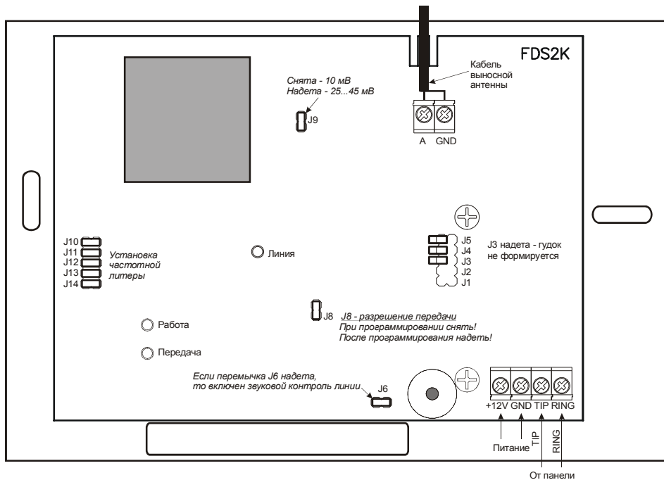
Рис. 2. Монтажная схема передатчика
