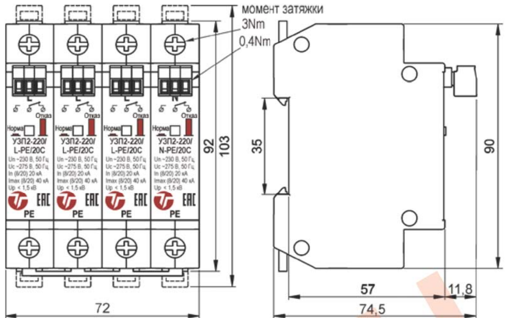
Рис.1 Габаритные размеры
