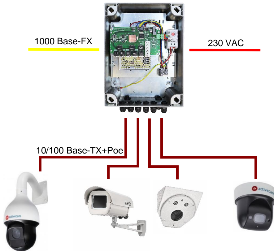
Рисунок 2. Типовые схемы подключения коммутаторов: Релион-SW-1G-1/4Poe+/60W; Релион-SW-1G-1/4Poe+/150W по оптическому кабелю.
