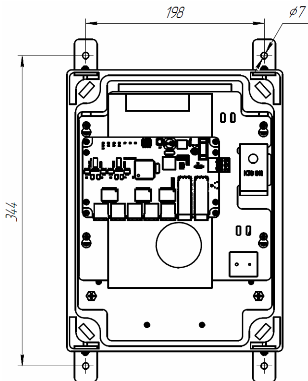
Рисунок 14. Расположение крепежных элементов коммутатора
