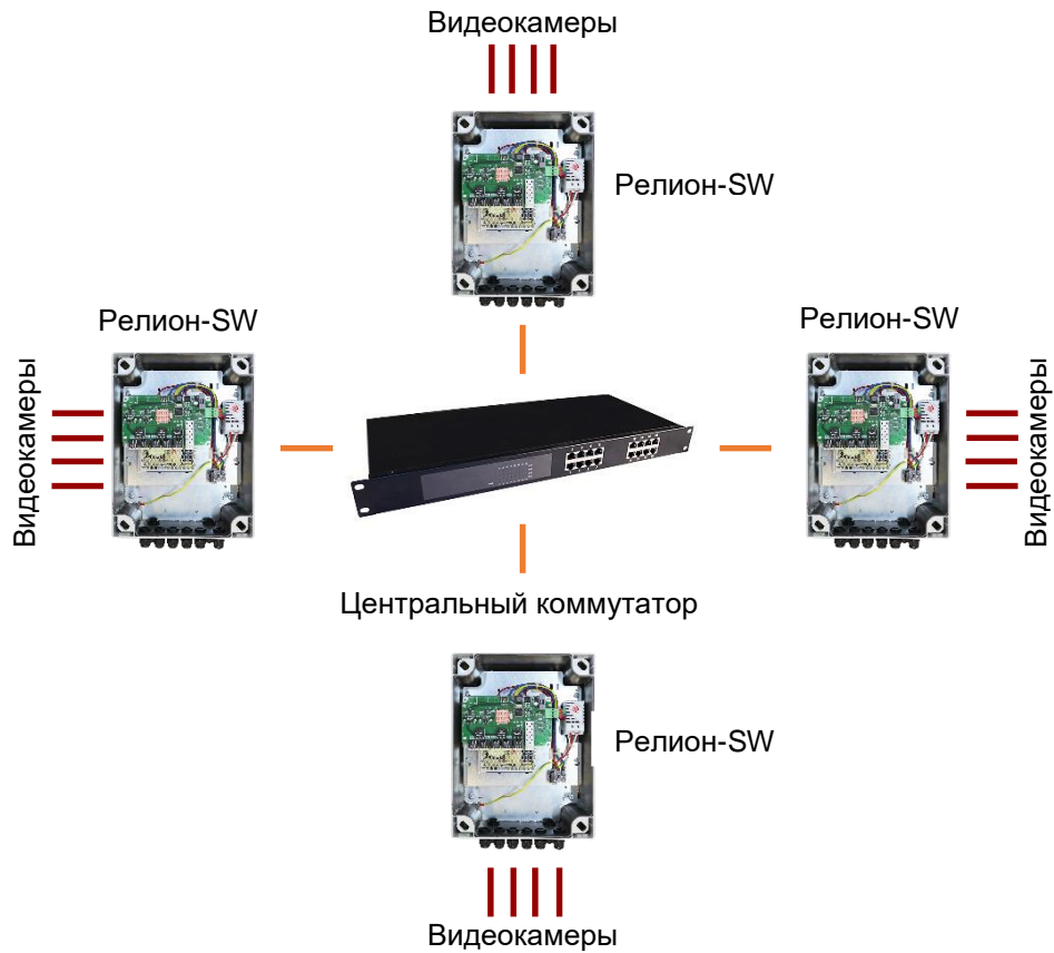
Рисунок 10. Подключение коммутаторов в топологию «звезда» по меди
