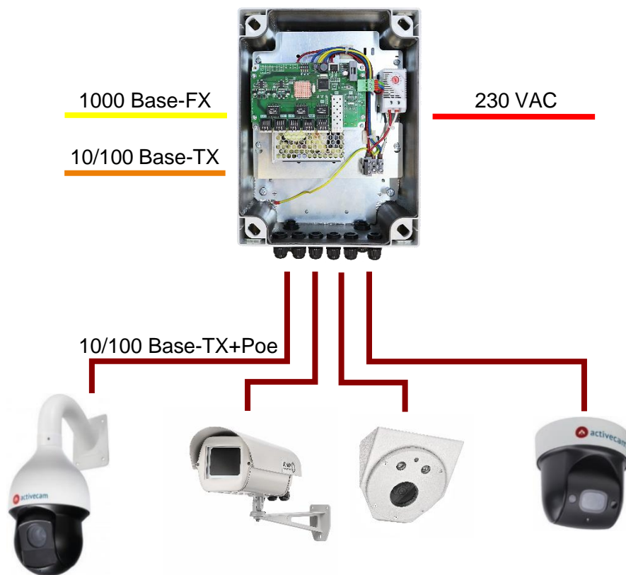
Рисунок 3. Типовая схема подключения коммутатора Релион-SW-1G-1/4Poe+/60W, Релион-SW-1G-1/4Poe+/150W по медному кабелю и оптическому кабелю.
