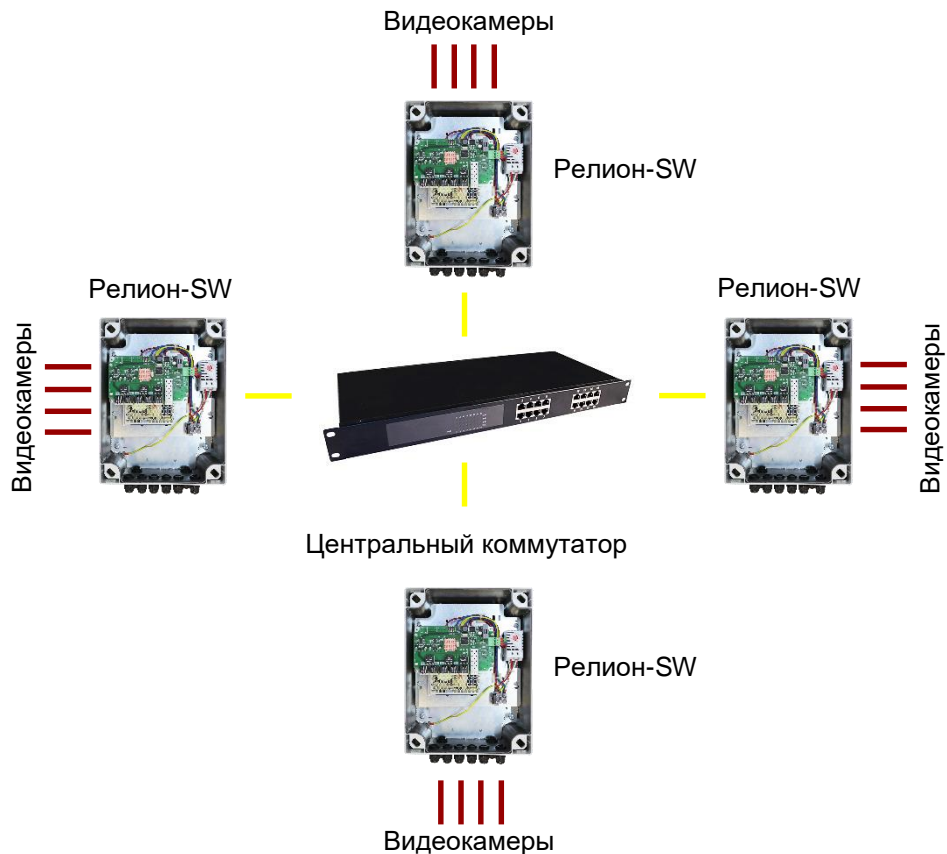
Рисунок 11. Подключение коммутаторов в топологию «звезда» по оптике
