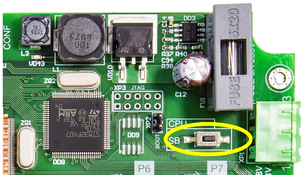
Рисунок 13. Кнопка сброса настроек коммутатора на заводские установки
