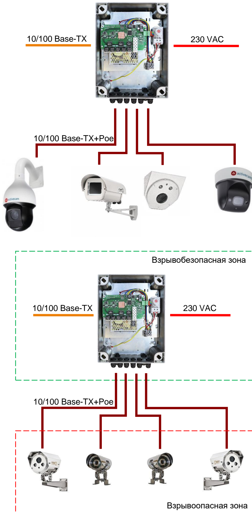
Рисунок 1. Типовые схемы подключения коммутаторов: Релион-SW-1G-1/4Poe+/60W; Релион-SW-1G-1/4Poe+/150W по медному кабелю.
