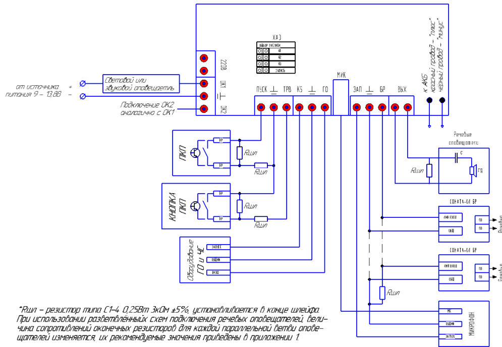
Рисунок 2. Схема внешних соединений прибора «С-КЛД»
