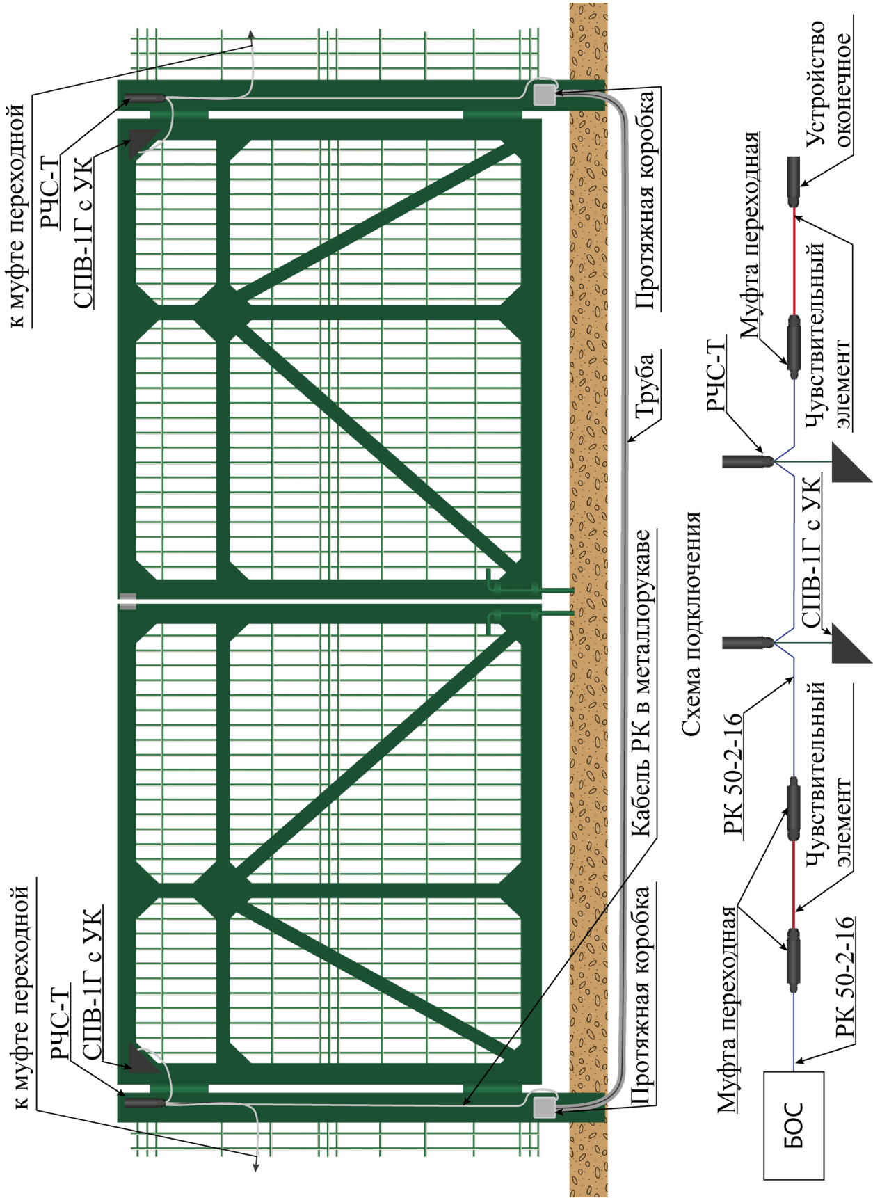
Рисунок 1.6– Организация охраны ворот (калитки) с использованием сен- сора СПВ-1Г с узлом крепления в единой зоне охраны периметра
