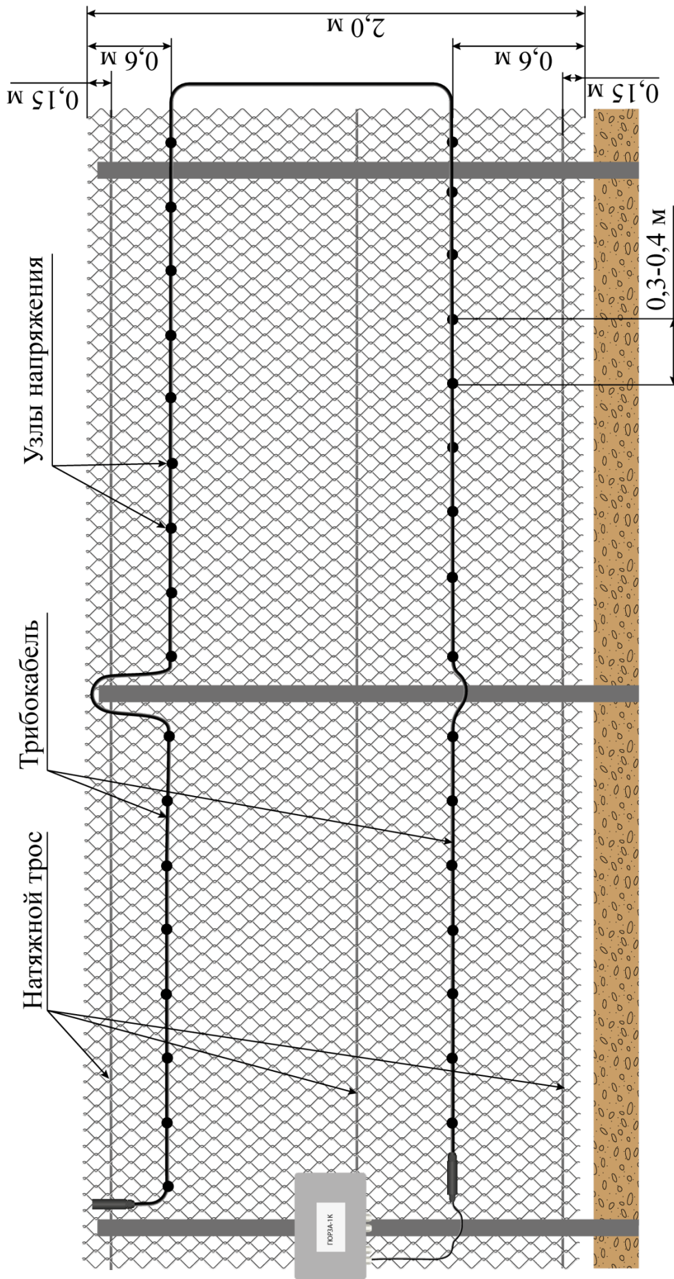
Длина зоны охраны до 250 м (Длина зоны охраны с ЧЭ ТППбэп-10П SKICHEL до 500 м)
