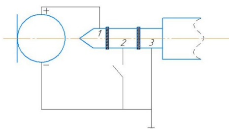
Рис.2. Внутренняя схема подключения
