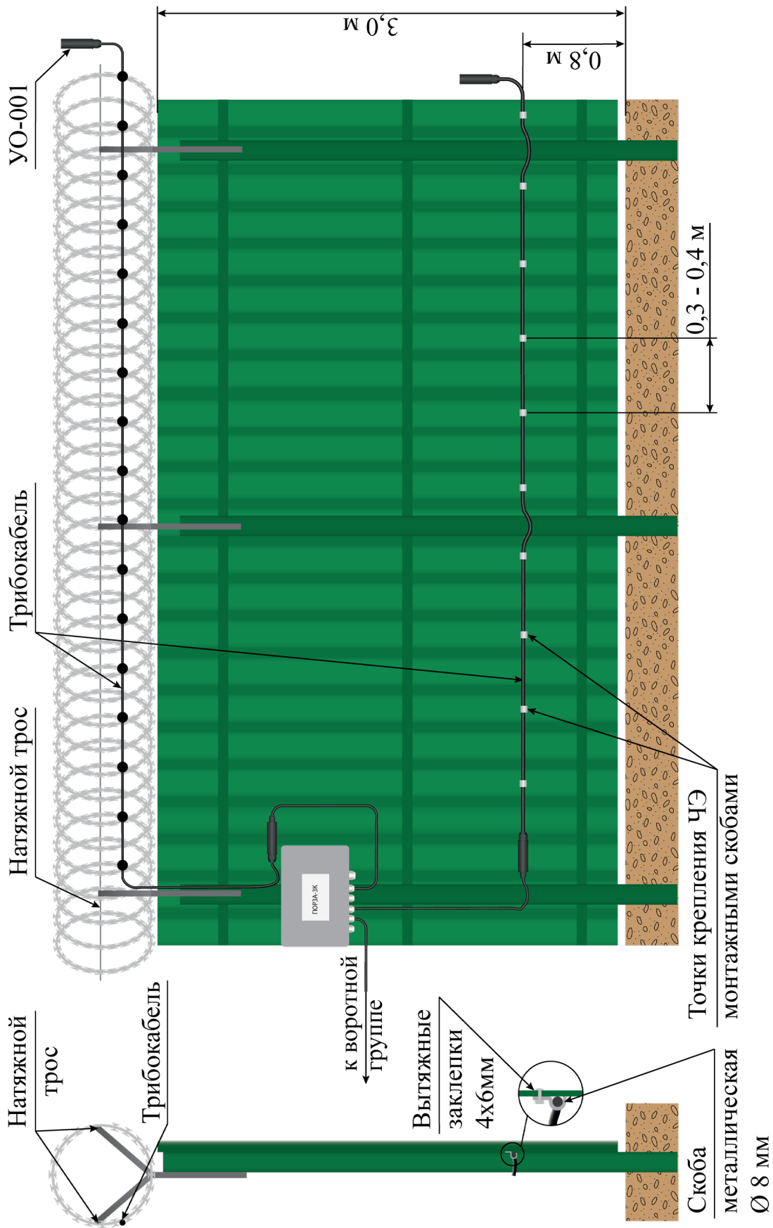
Длина зоны охраны до 500 м (Длина зоны охраны с ЧЭ ТППбэл-10П SKISHEL до 1000 м) Рисунок 1.2 – Вариант прокладки ЧЭ на ограждении из профлиста с козырьком из объемной спирали АКЛ
