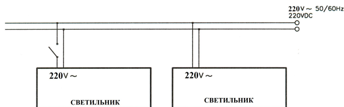
Рис. IV Схема подключения светильников для централизованных систем питания.
