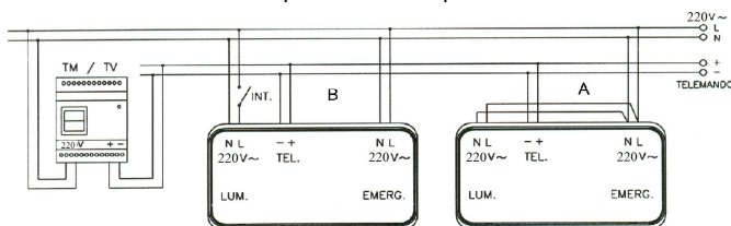
Рис. II - Схема подключения светильников с люминесцентными лампами постоянного типа работы
