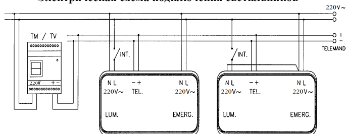
Рис. I - Схема подключения светильников с люминесцентными лампами комбинированного типа работы
