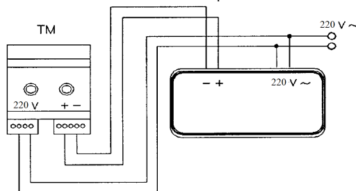
Рис. II - Схема подключения светильников с люминесцентными лампами постоянного типа работы
