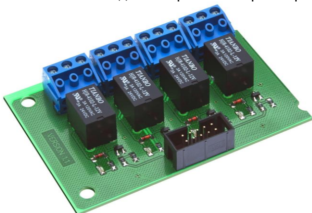
Рисунок 1. Релейный расширитель
