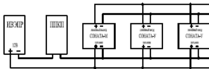
Схема подключения одного оповещателя охранно-пожарного речевого "SONATA-M" с одним и более оповещателями "SONATA-Y"
