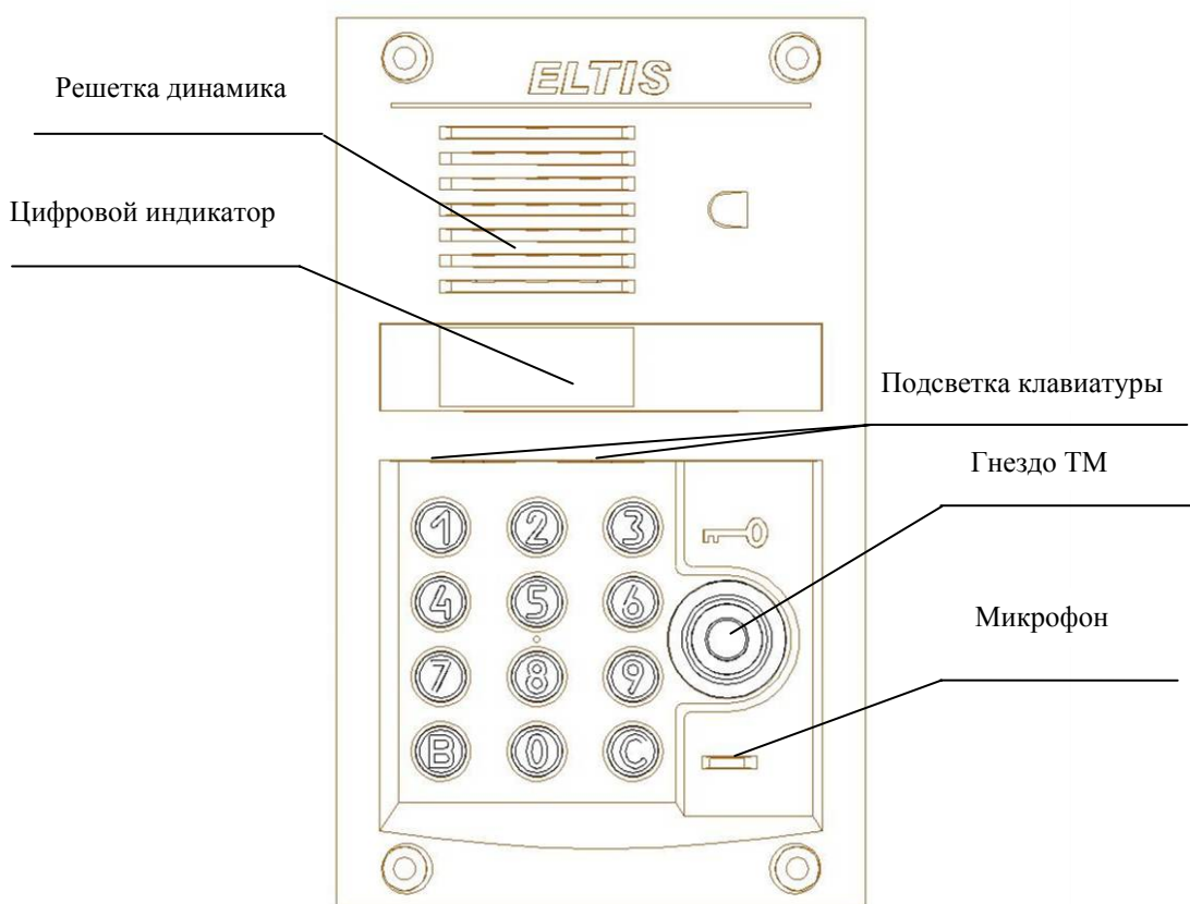
Рис.1 Внешний вид со стороны лицевой панели блока вызова DP400-TD22.
