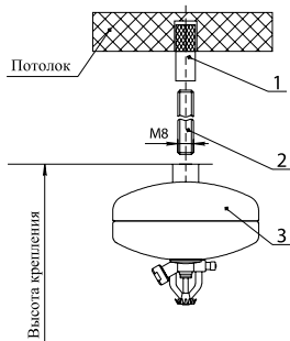
Рисунок 4 — Схема крепления модуля к потолку на подвесной конструкции
