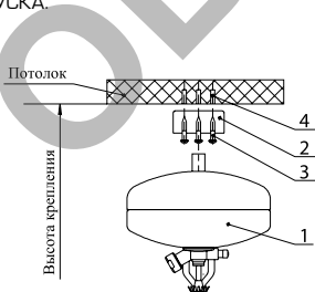
Рисунок 3 — Схема крепления модуля к потолку
