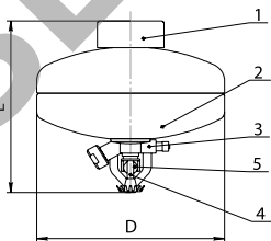
Рисунок 1 — Устройство модулей МПП«МИГ» А 1 – подвеска, 2 – корпус, 3 – запорно-пусковое устройство, 4 – тепловой замок. 5 – устройство электрозапуска
