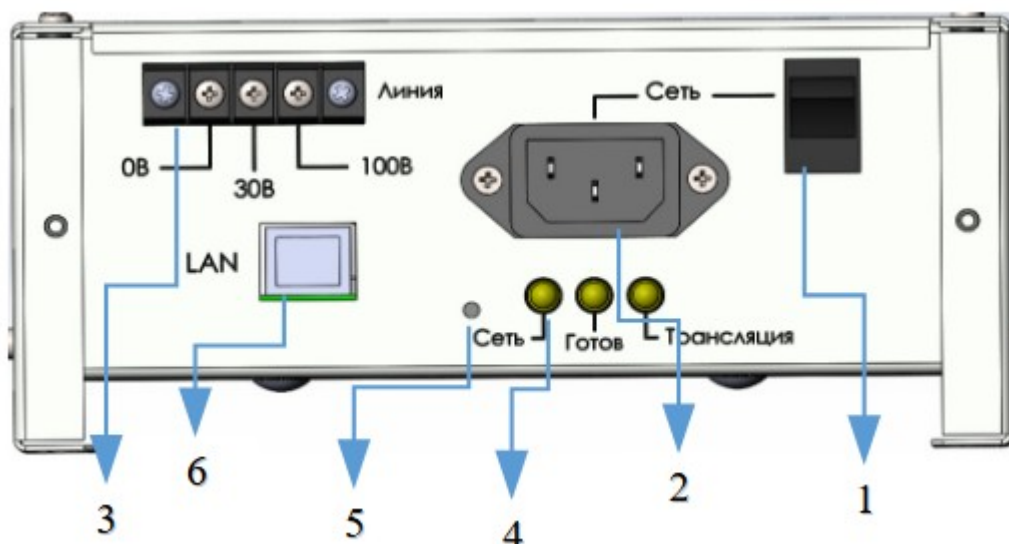
Рисунок 2 - Коммутационный отсек, вид снизу
