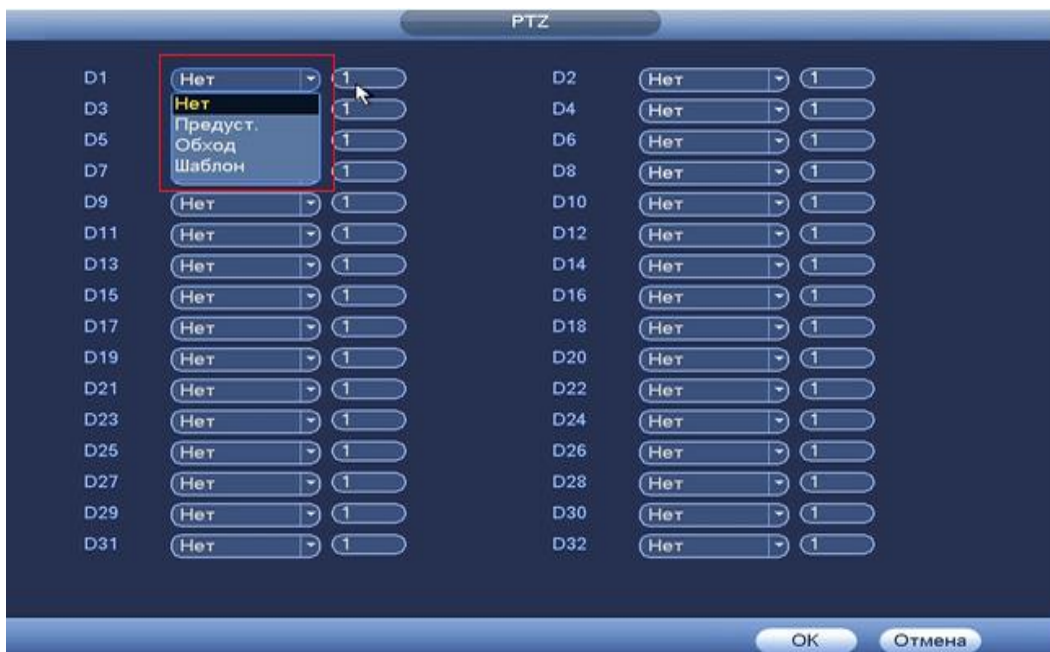
Рисунок 8.3.3.5.4 Установка предустановок.
