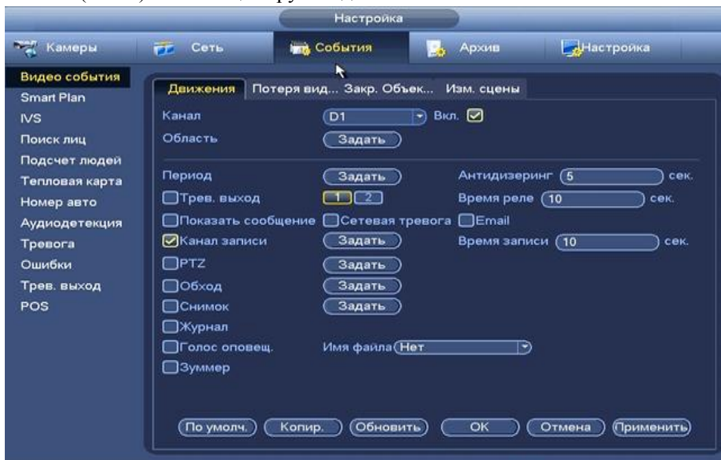
Рисунок 8.3.3.1.1.6 Установка настроек
