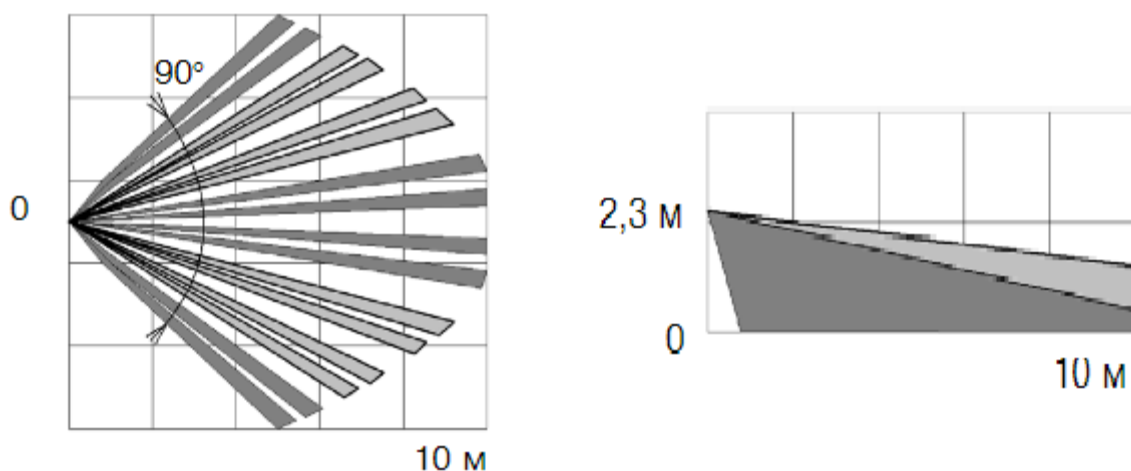
Рисунок 2.4 Зона обнаружения
