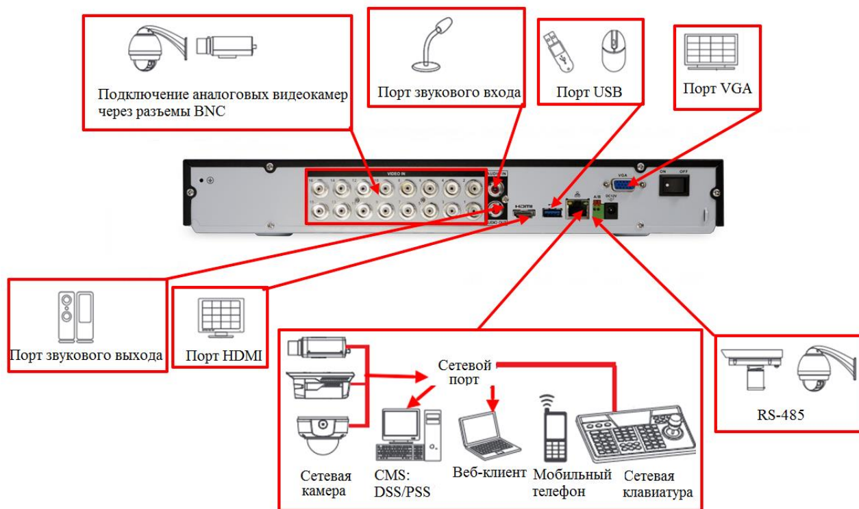
Рисунок 4.2 Внешний вид задней панели
