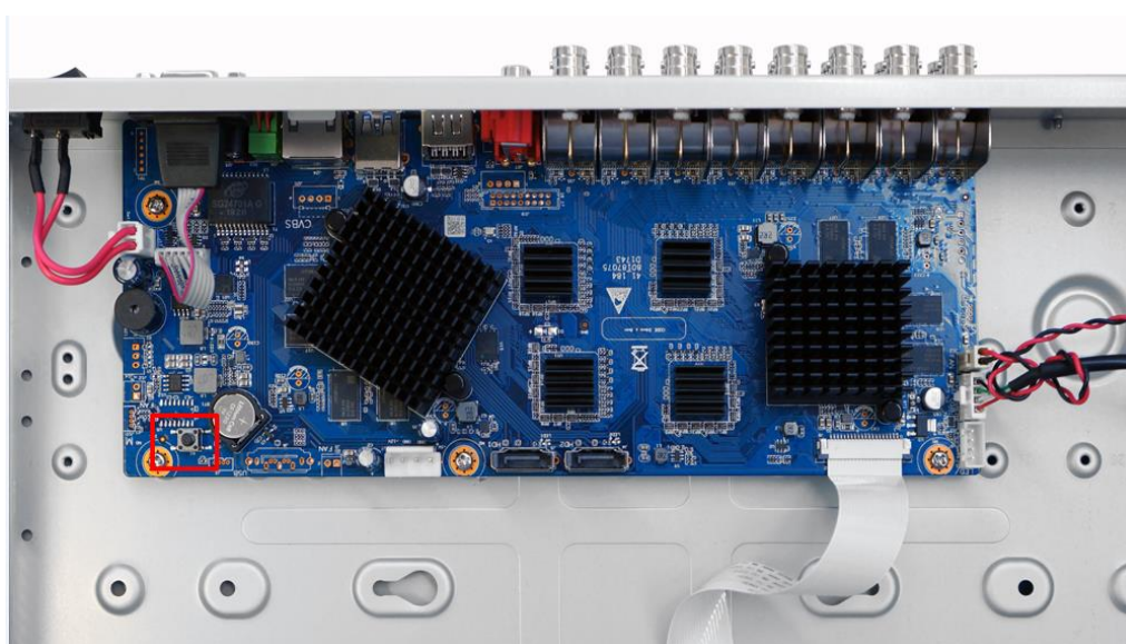
Рисунок 8.124 Кнопка сброса на плате
