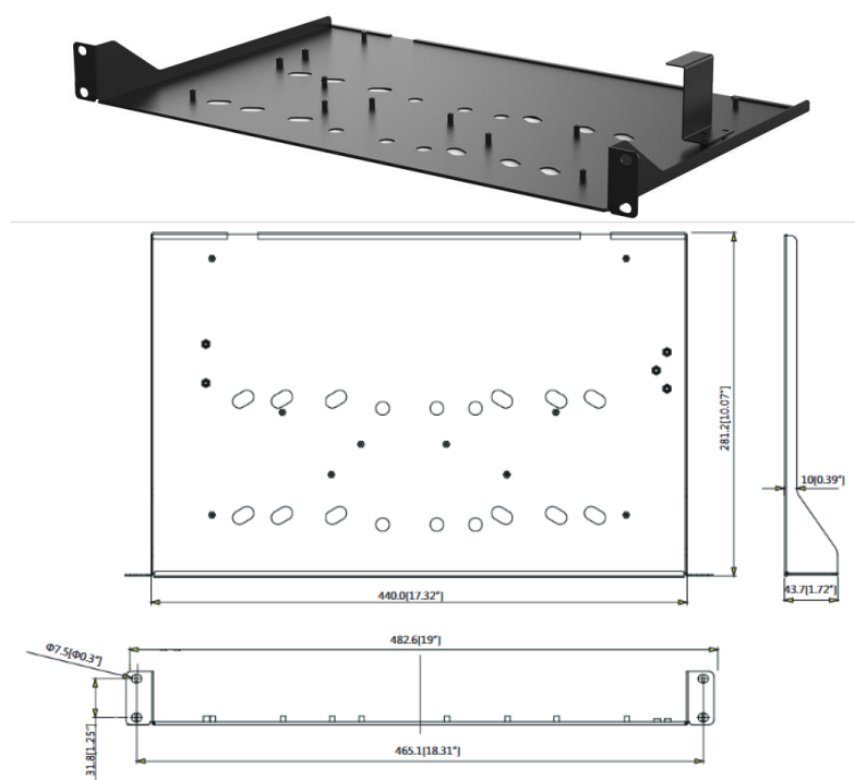
Рисунок 5.2 Внешний вид и габариты BR-111
