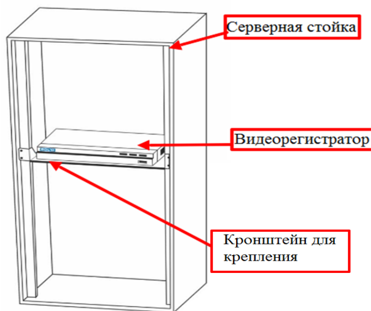
Рисунок 5.3 Монтаж видеорегистратора в 19"-стойку с помощью кронштейна
