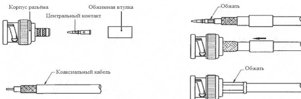
Рисунок 5.1 Схема обжима BNC
