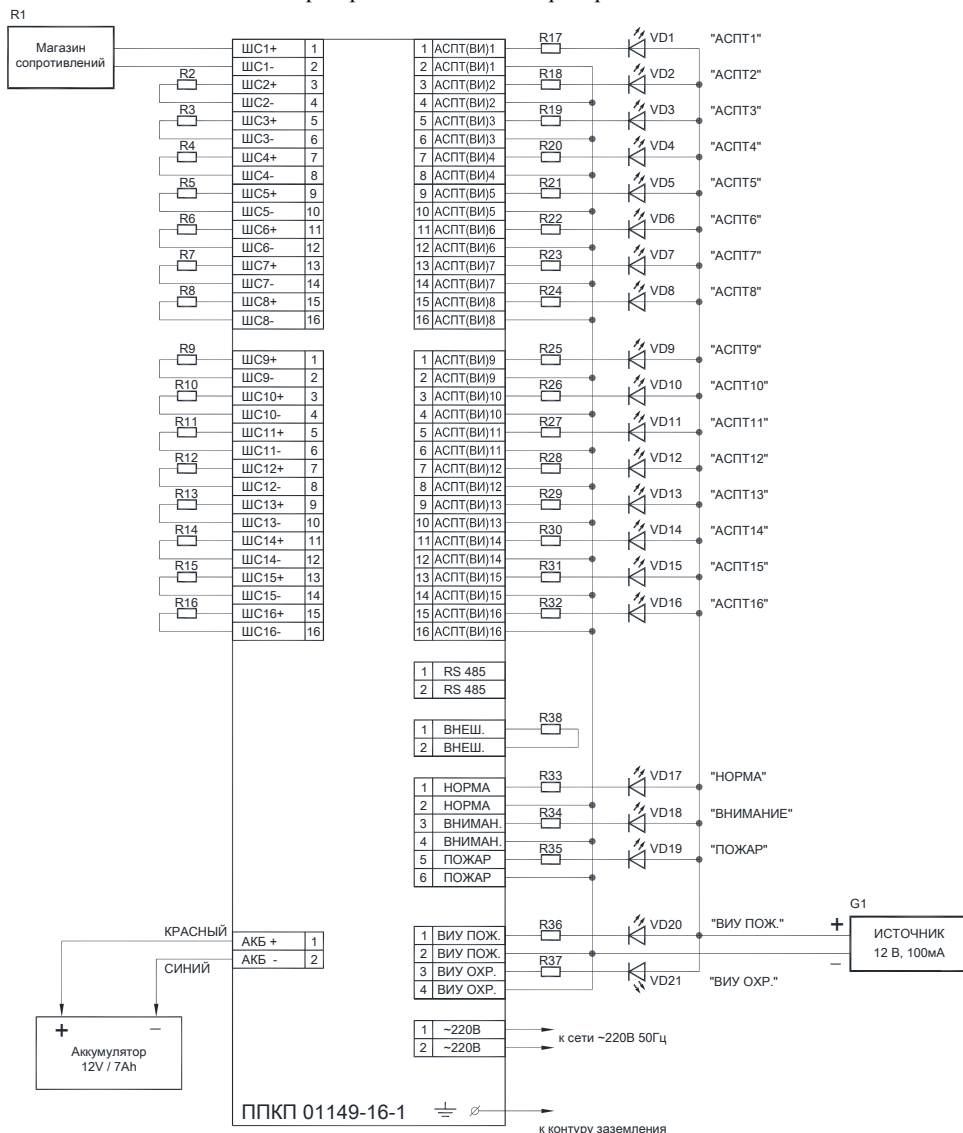
Схема внешних подключений прибора ППКП01149-16-1 «ЯХОНТ-16И» при проведении общей проверки.
