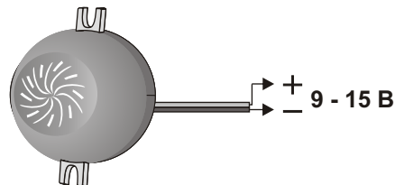
Рис.2 Схема подключения ПКИ-МБ.
