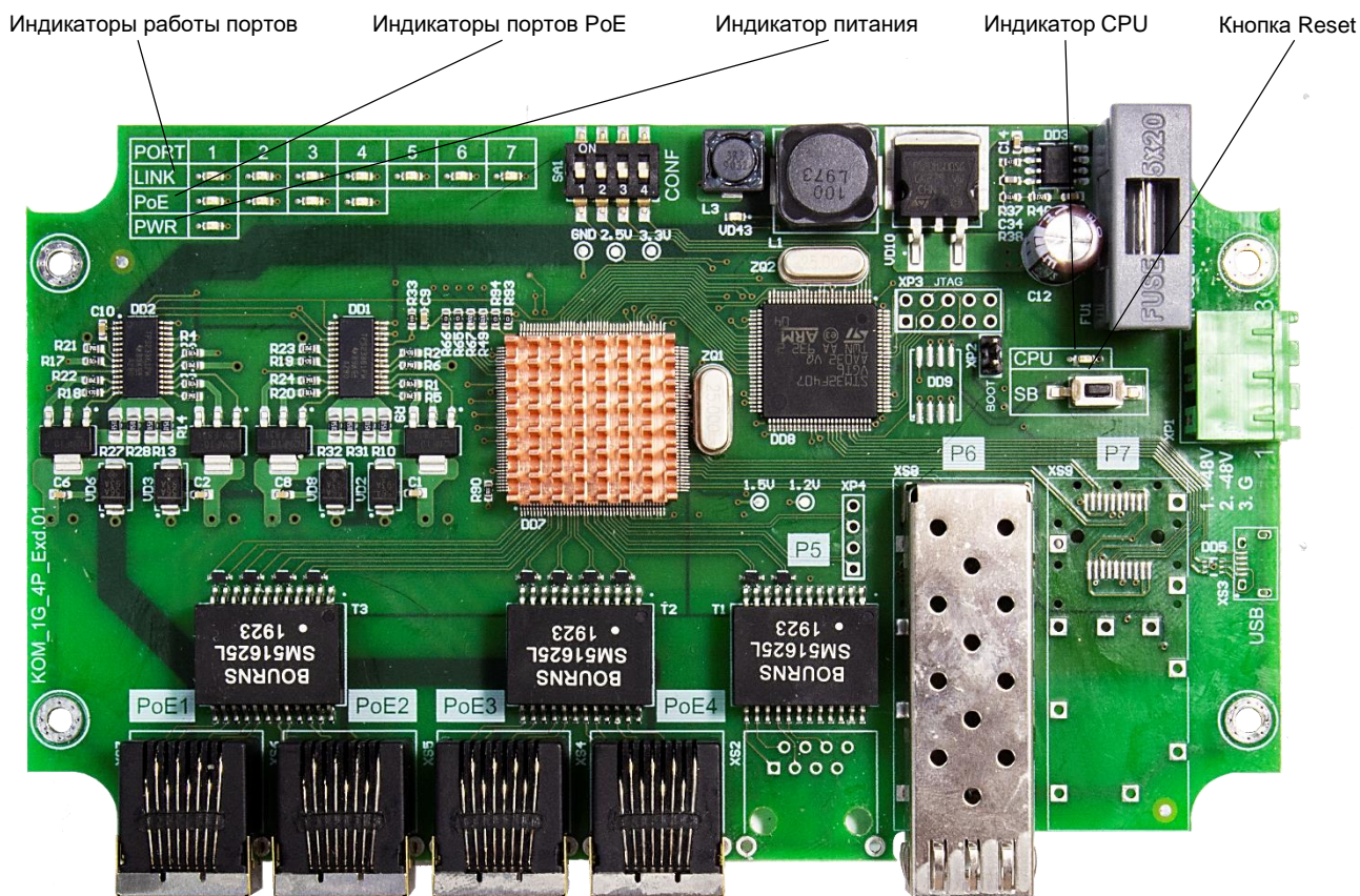
Рис. 4. Расположение элементов Релион-SW-1G-4Poe+/150W
