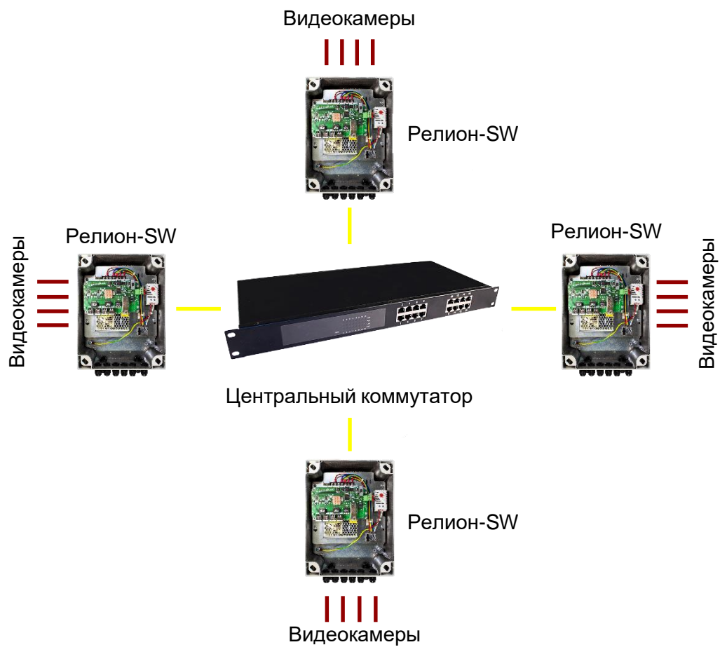
Рисунок 7. Подключение коммутаторов в топологию «звезда»
