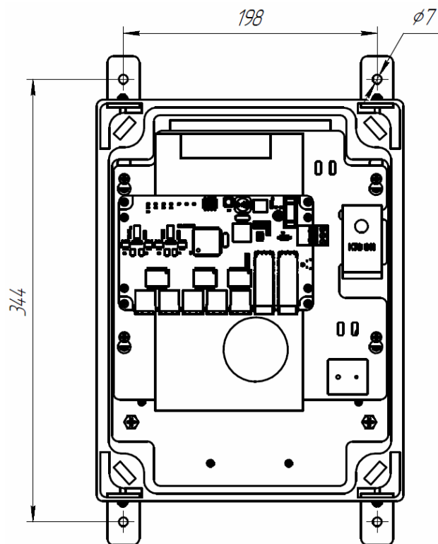
Рисунок 10. Расположение крепежных элементов коммутатора
