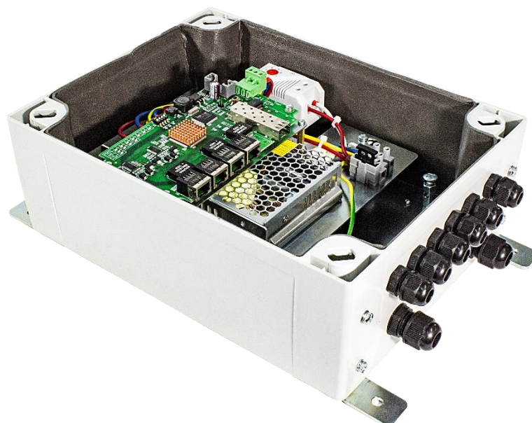
Рисунок 3. Релион-SW-1G-4Poe+/150W вид изнутри
