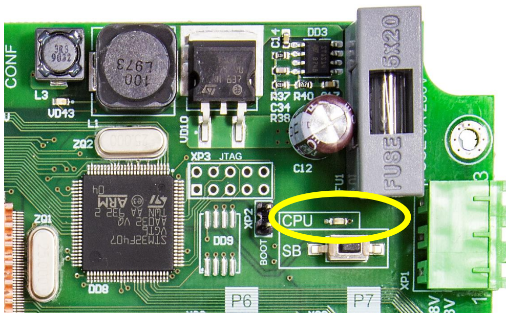
Рисунок 8. Расположение элементов индикации и настройки на плате коммутатора
