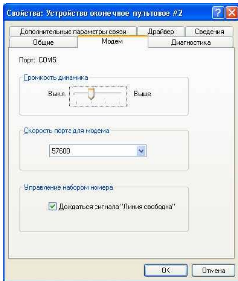
Рис. 6. Свойства назначенного СОМ-порта
