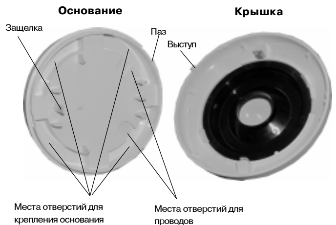
Рис. 2. Основание и крышка извещателя
