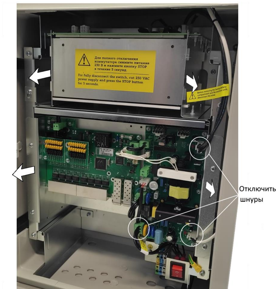
Рис. 7.1.1. Извлечение отсека АКБ и электронного узла
