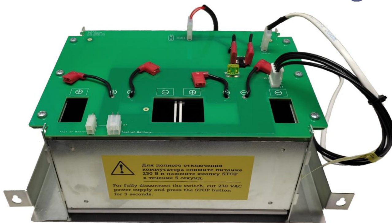
Рисунок 3.6.1 – отсек АКБ
