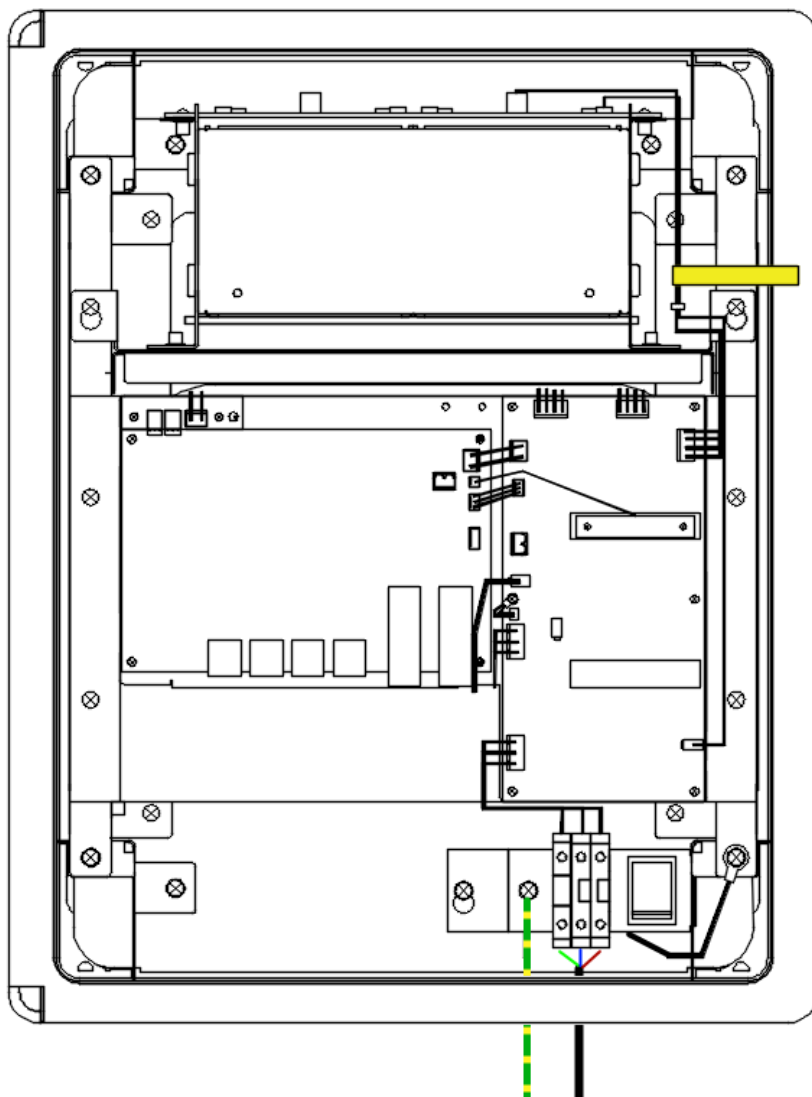
Рисунок 7.7.1 - Схема подключения коммутатора.
