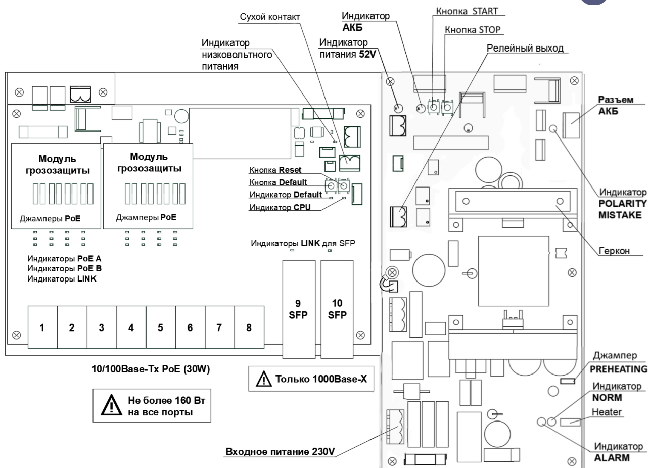
Рисунок 3.4.2 – Расположение элементов PSW-2G8F+UPS-Box
