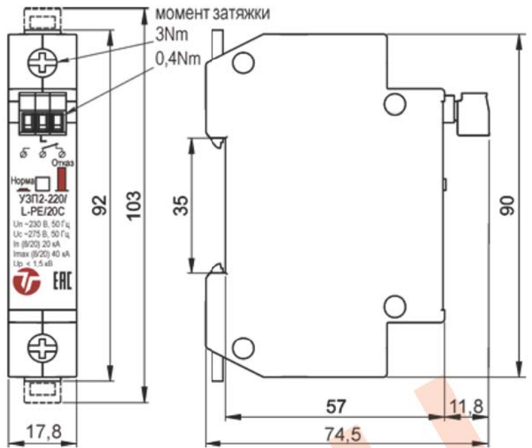
Рис.1 Габаритные размеры
