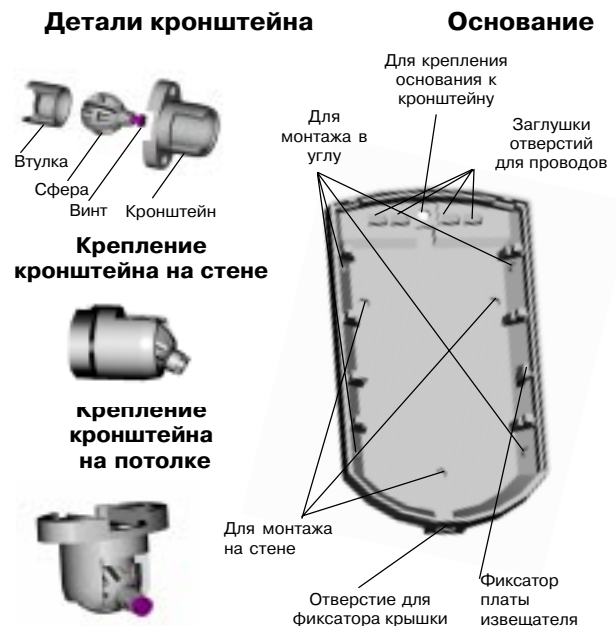
Рис. 1. Основание извещателя и кронштейн
