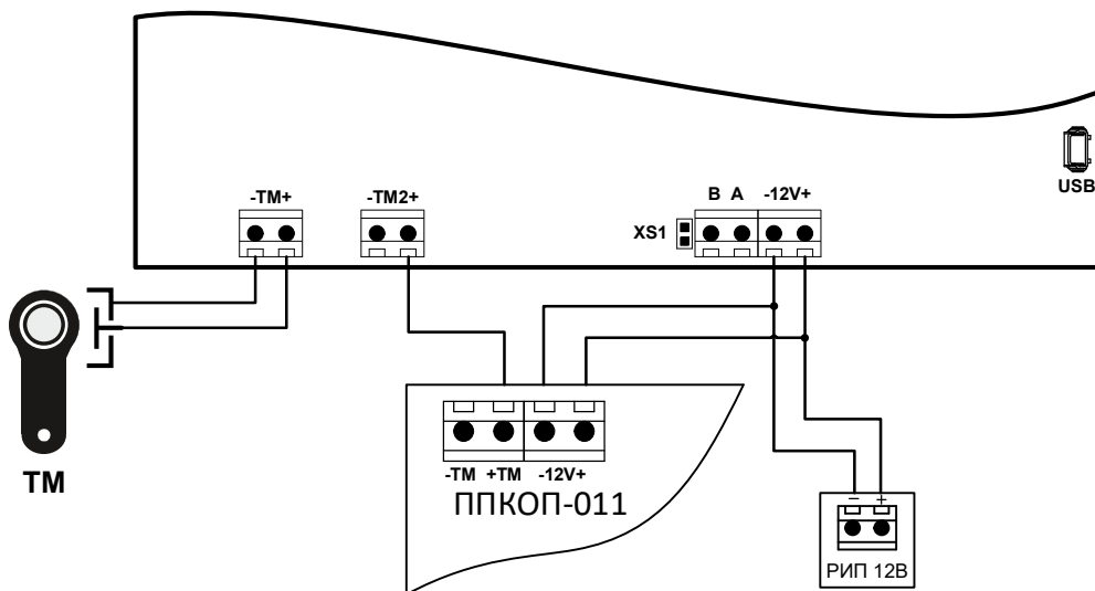
Рисунок 9 – Схема подключения клавиатуры к приборам серии ППКОП-011 в режиме ТМ
