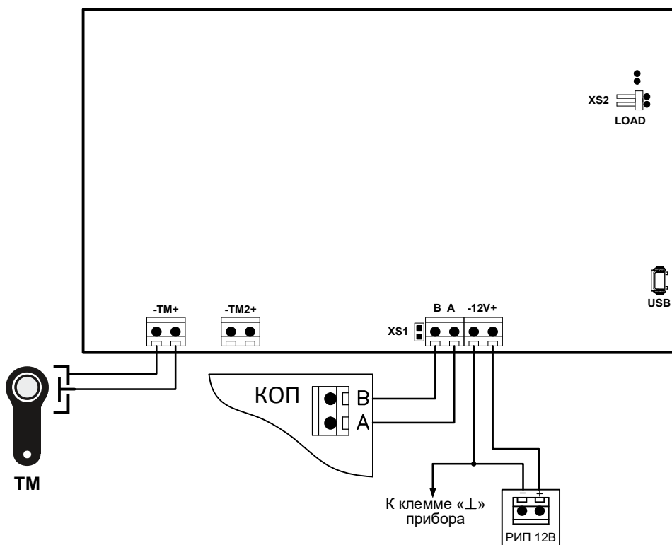
Рисунок 8 – Схема подключения клавиатуры к приборам серии Приток-А-КОП по ШР
