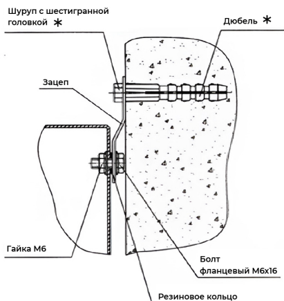
Рисунок 2 - Установка на стену на зацепках
