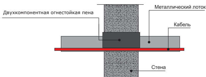
Монтаж проходки из двухкомпонентной огнестойкой пены для металлического кабельного лотка
