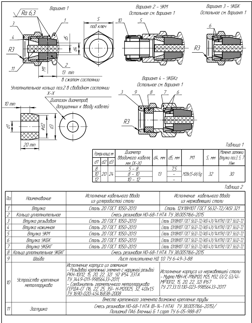
Рисунок В.3 – Чертеж средств взрывозащиты кабельных вводов
