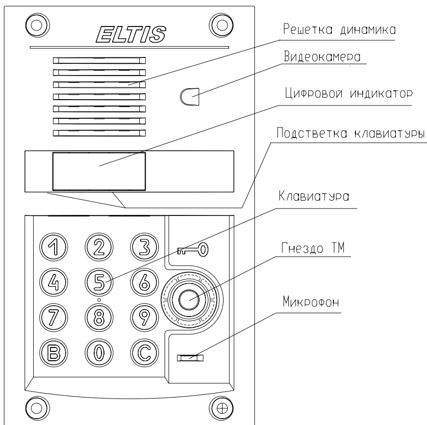
Рис.1 Внешний вид со стороны лицевой панели блока вызова DP303-TDV22.
