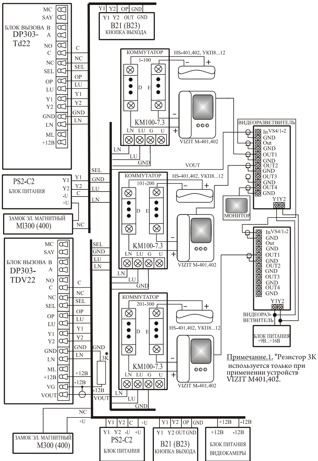
Рис.3 Пример схемы подключения DP303-TDV22 в составе домофонного комплекса.
