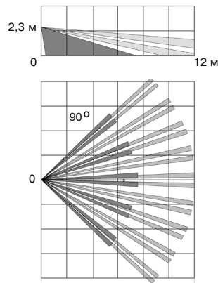
Рисунок 1 – Диаграмма зоны обнаружения
