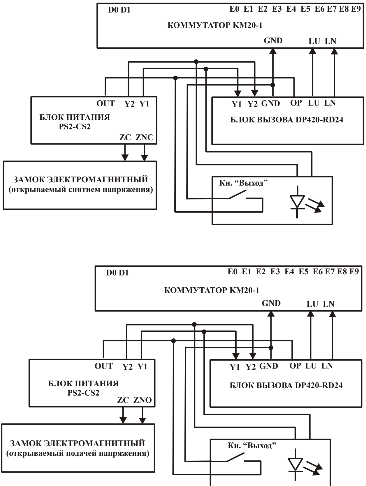
Рис.4 Схемы подключения различных типов замков, не имеющих собственной схемы управления.
