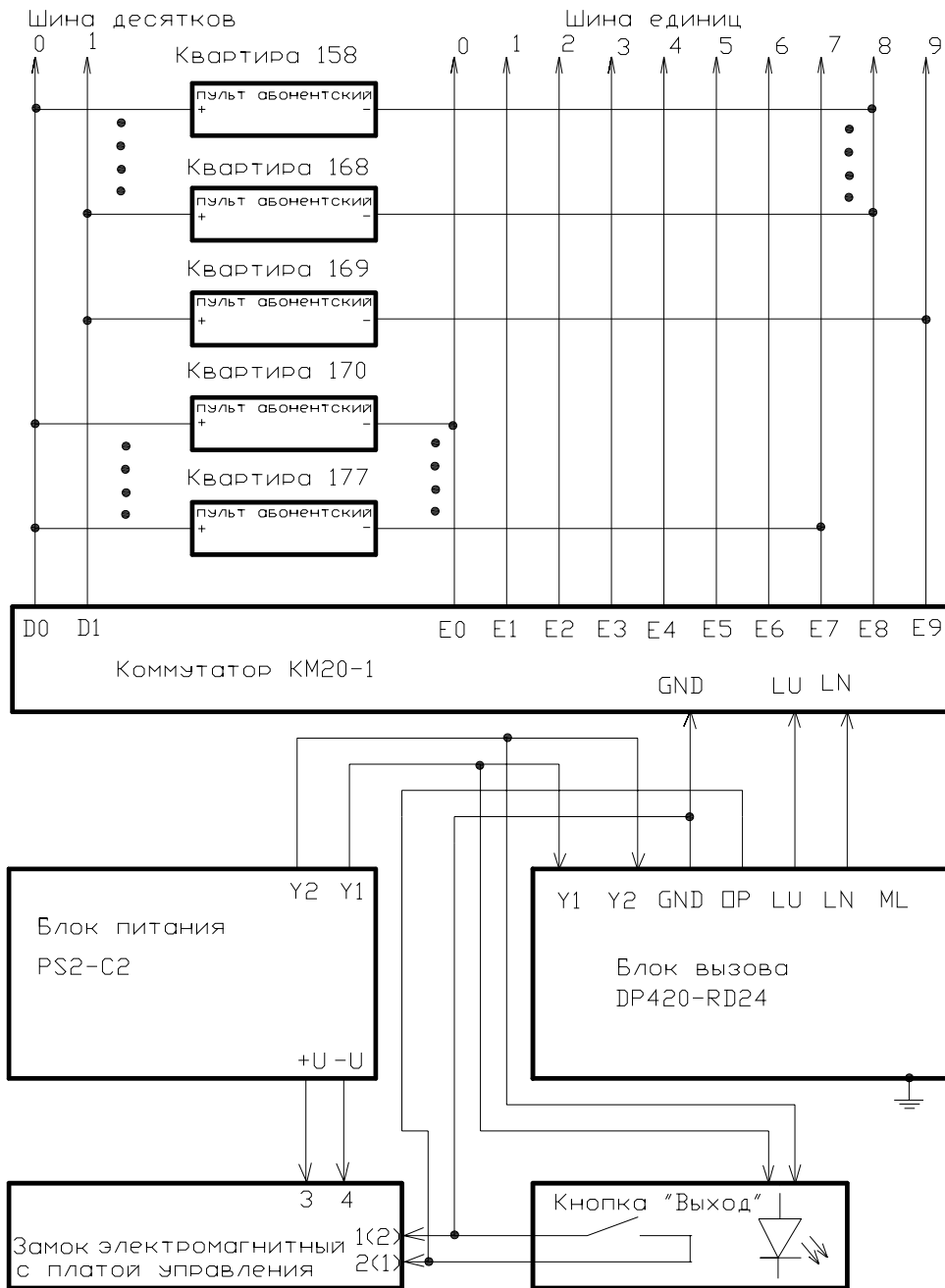
Рис. 3 Монтажная схема соединения блоков домофонного комплекса.
