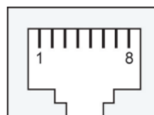
8-контактный RJ45
