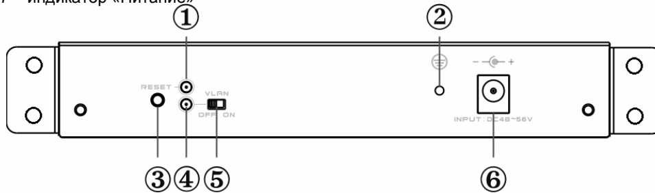
Рисунок 5 – задняя панель коммутатора**
