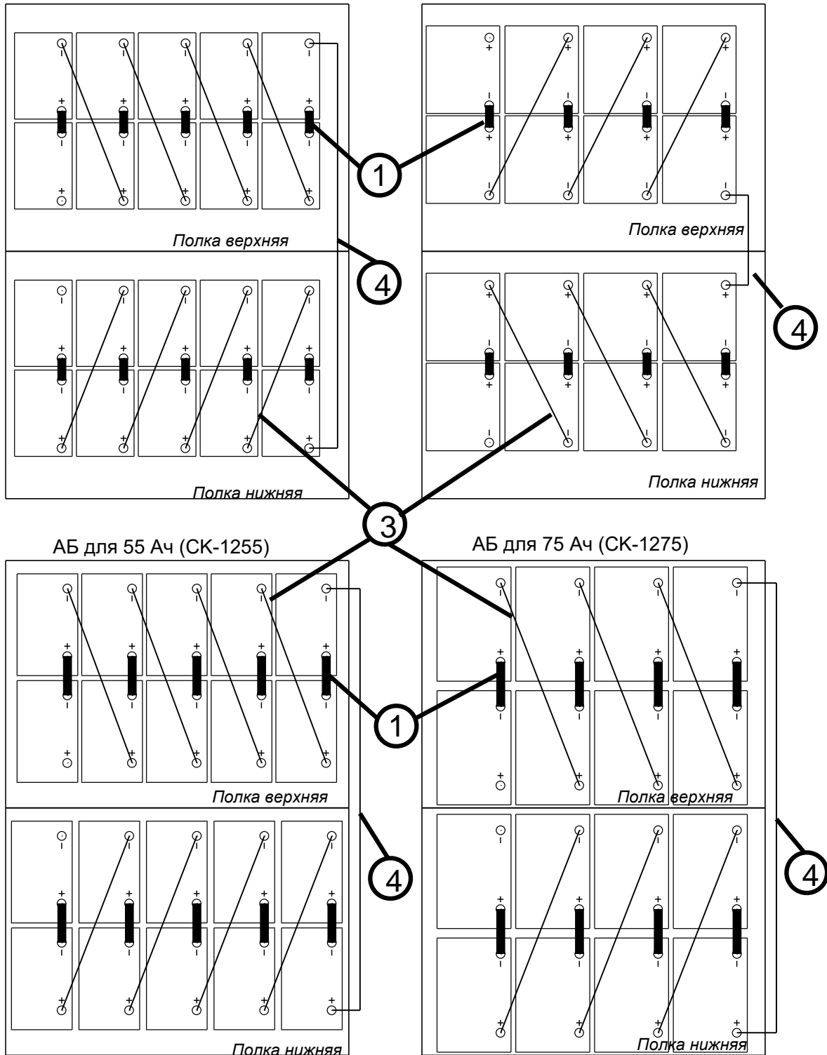
Типовое расположение АБ в стеллаже типа MBS-04 АБ для 33 Ач (СК-1233) АБ для 40 Ач (СК-1240)
