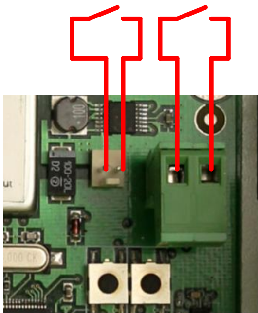
Рисунок 3.6 - Сухие контакты
