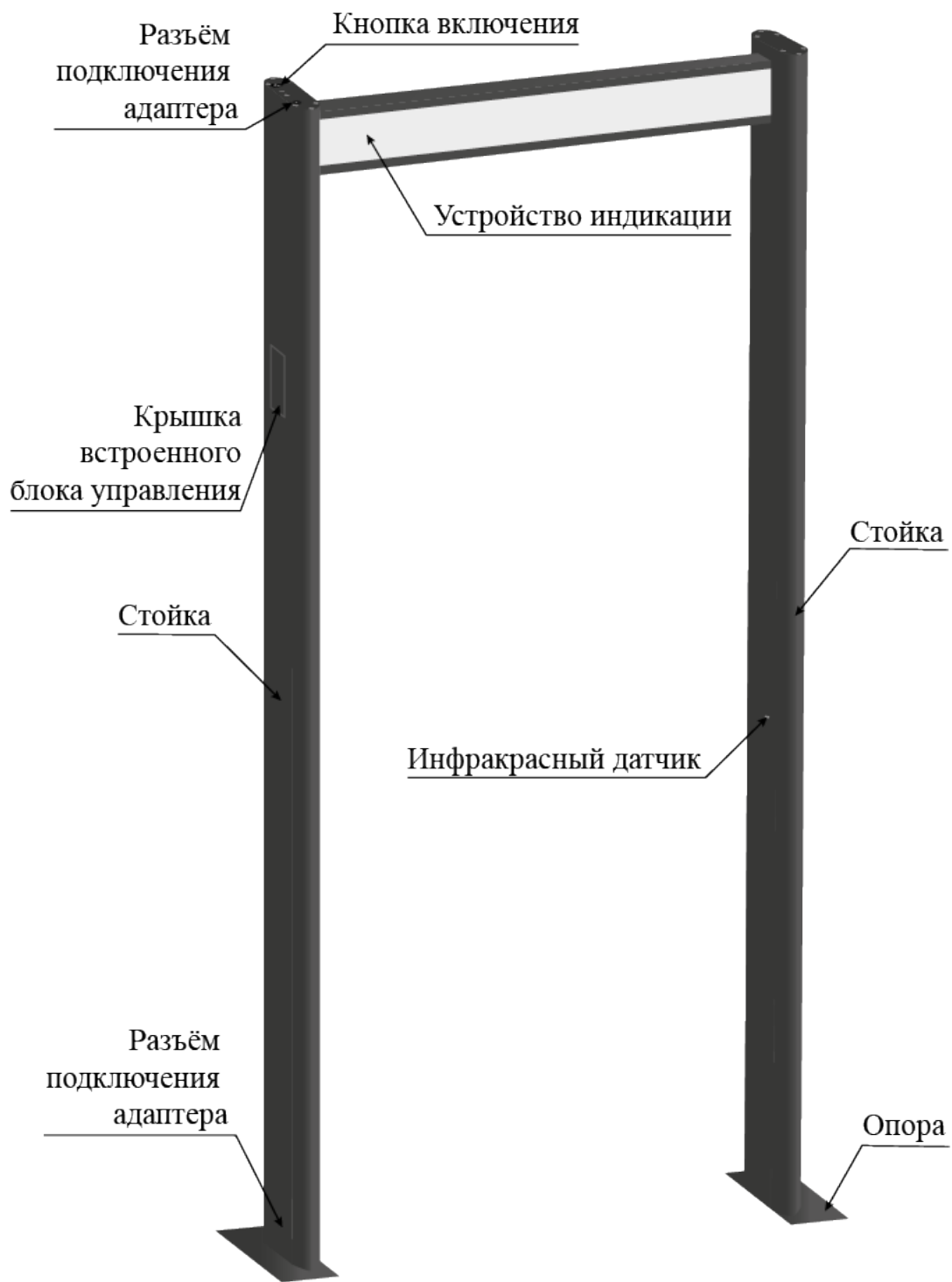
Рисунок 1.1 – Общий вид металлодетектора
