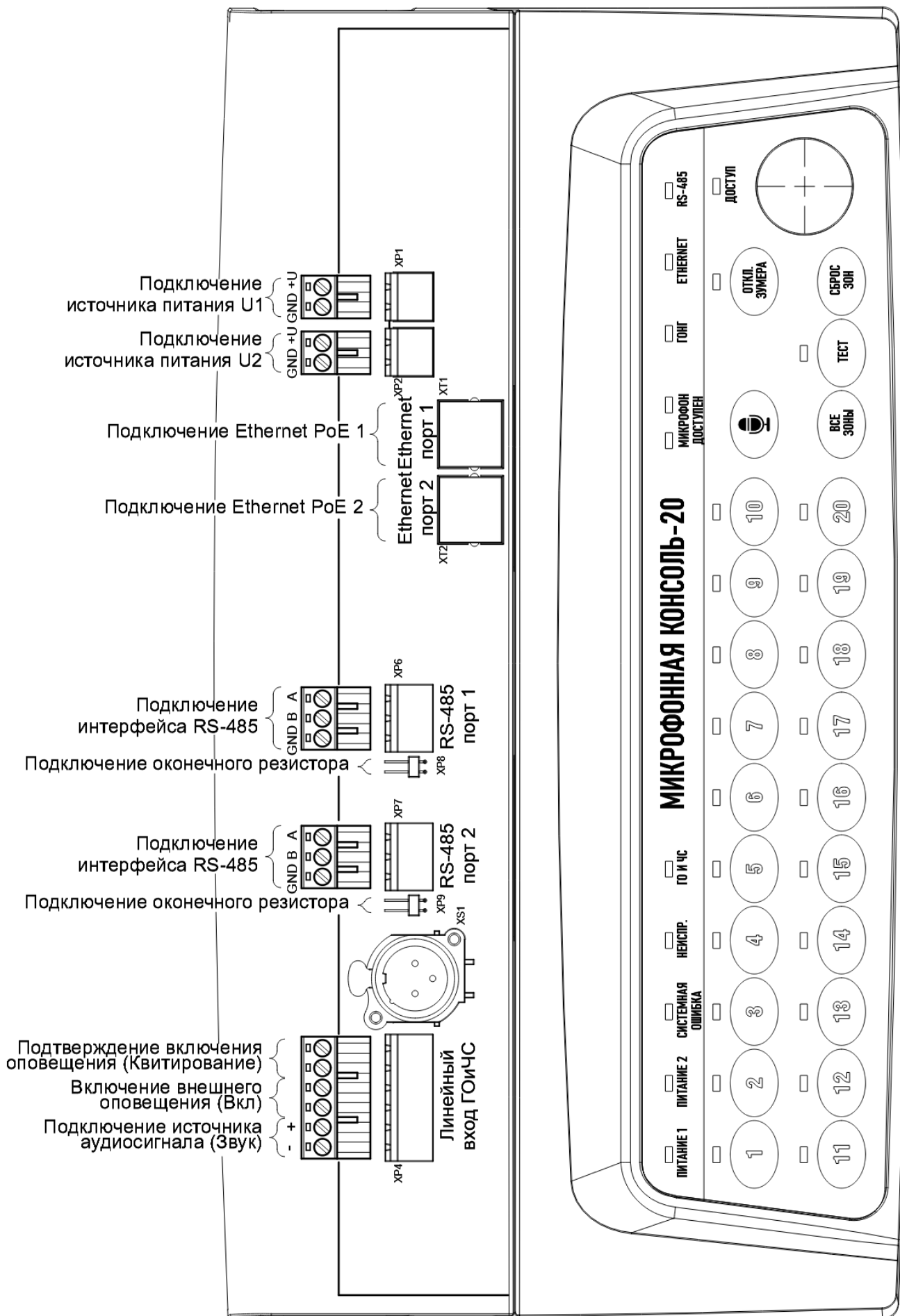
Рисунок 2.2.6. Схема подключения консоли.
