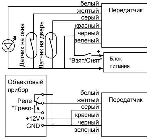
Рис. 2. Примеры монтажа передатчика
