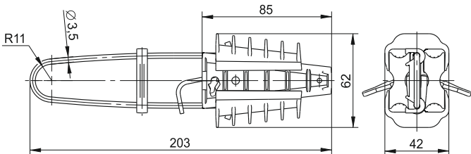
Габаритные размеры
