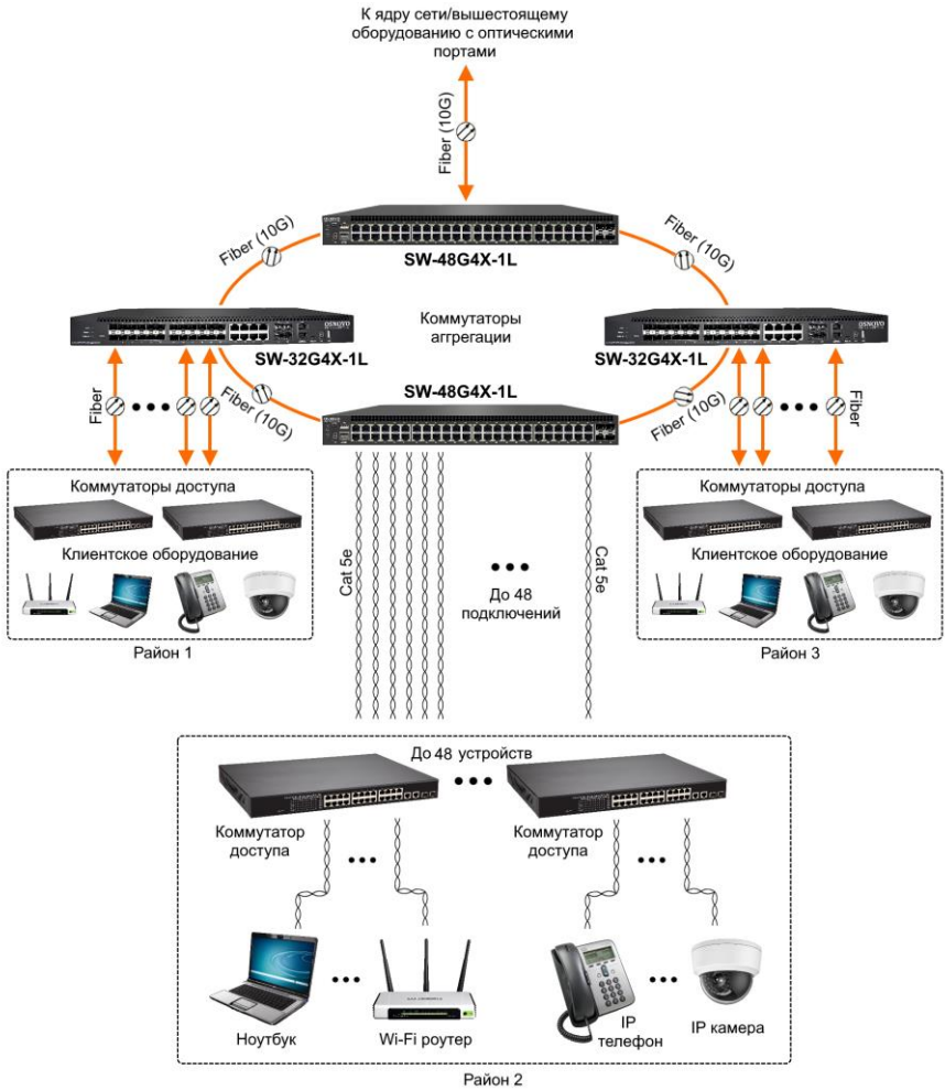
Рис. 4 Схема подключения коммутатора SW-48G4X-1L на примере построения сети оператора связи
