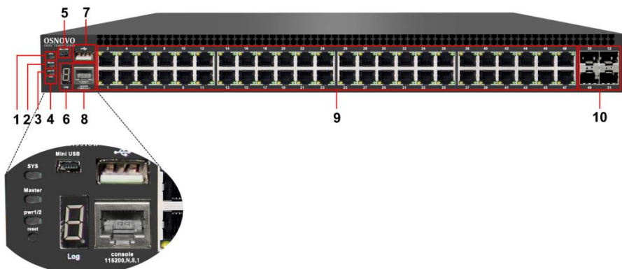
Рис.2 Коммутатор SW-48G4X-1L, разъемы, кнопки и индикаторы на передней панели
