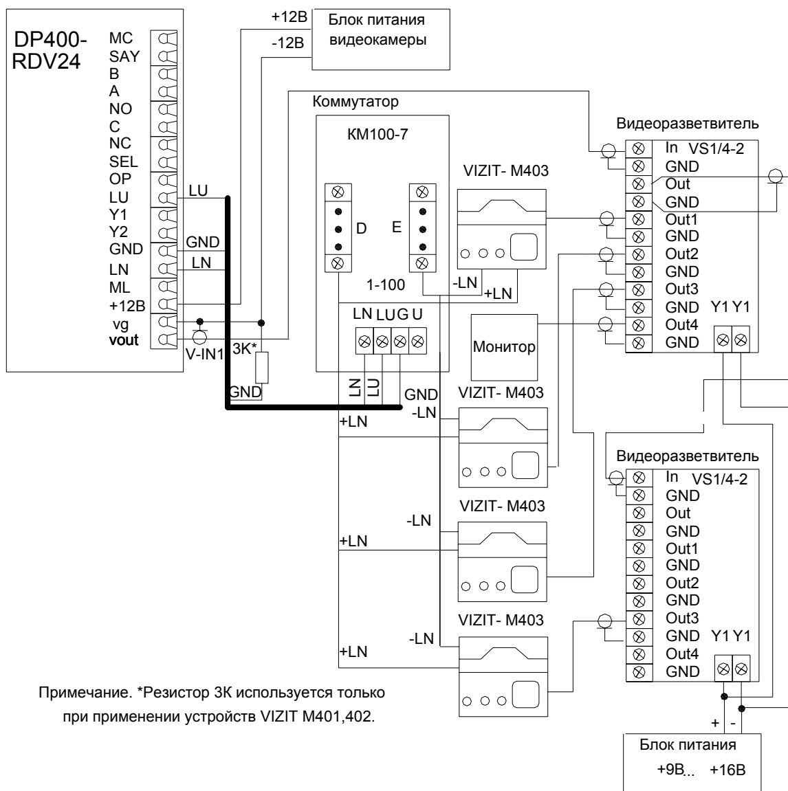
Рис.5 Схема подключения видеоканала блока вызова DP400-RDV24. (Пример с двумя видеоразветвителями)
