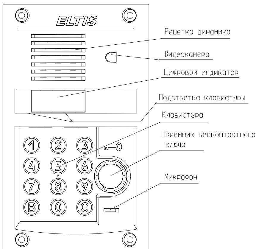
Рис.1 Внешний вид со стороны лицевой панели блока вызова DP400-RD24 Примечание. Видеокамера устанавливается для исполнения DP400-RDV24.
