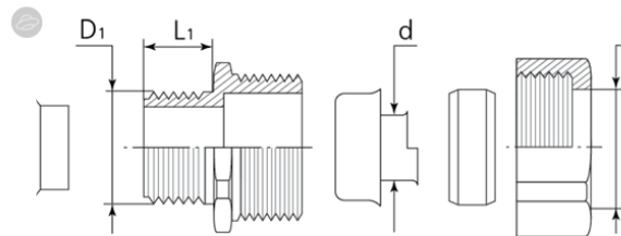
Приложение 2 – Последовательность сборки вводного узла оповещателей
