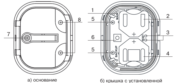
Рисунок 2 – Конструкция извещателя
