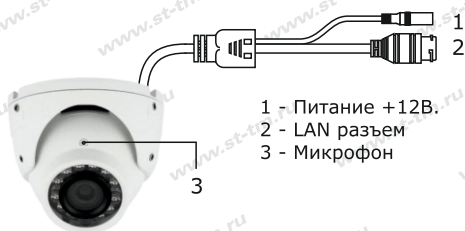
Рис. 1 Схема подключения видеокамеры
